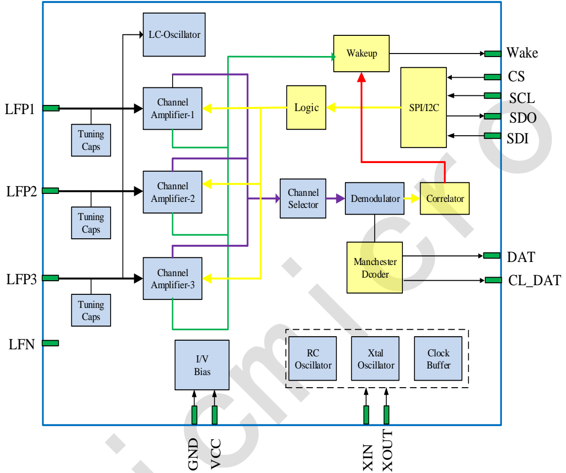
图 2-1：功能框图
