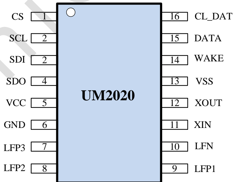
图 3-2: TSSOP16 封装管脚分布图
