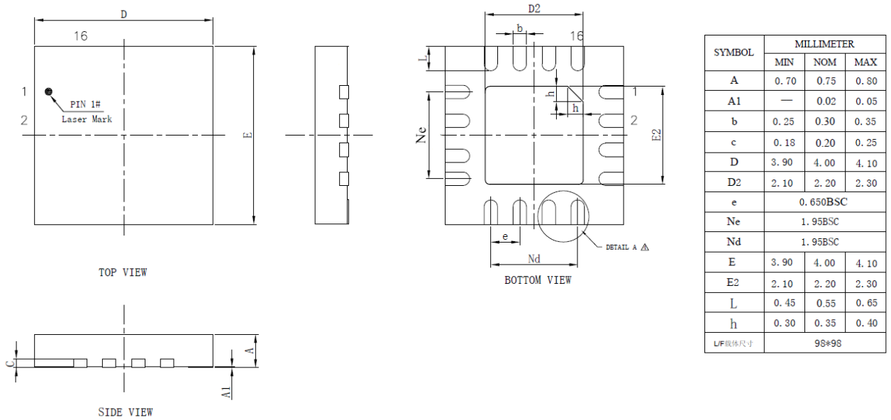
图 6-1: QFN16 封装图
