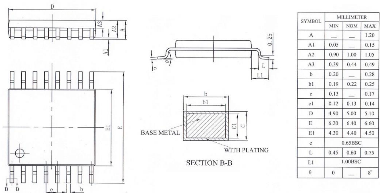
图 6-2: TSSOP16 封装图
