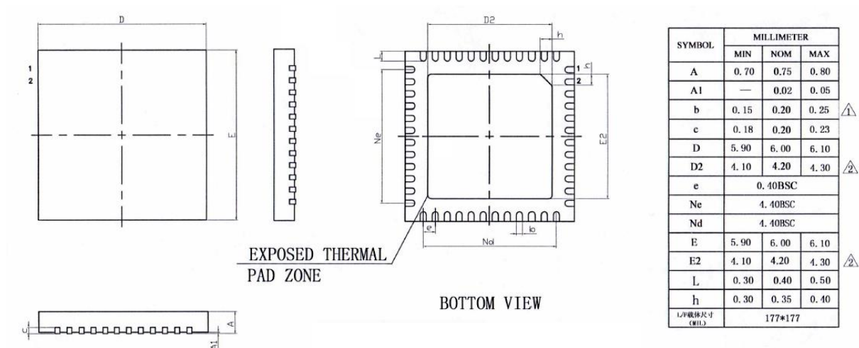
图 5-5: QFN48 封装尺寸图
