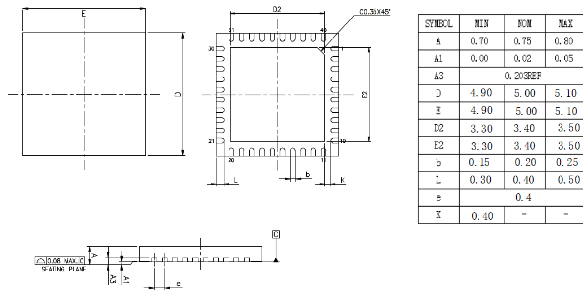
图 5-6: QFN40 封装尺寸图
