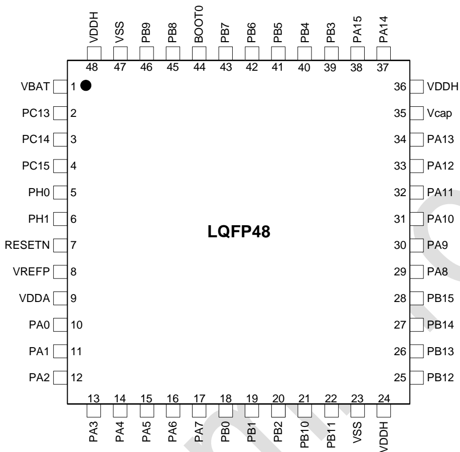
图 3-5: LQFP48 引脚分布图
