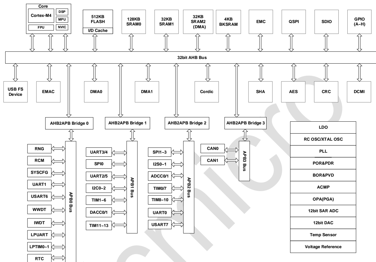
图 1-1：功能框图
