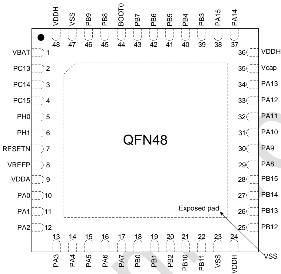
图 3-6: QFN48 引脚分布图
