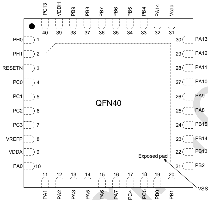
图 3-7: QFN40 引脚分布图
