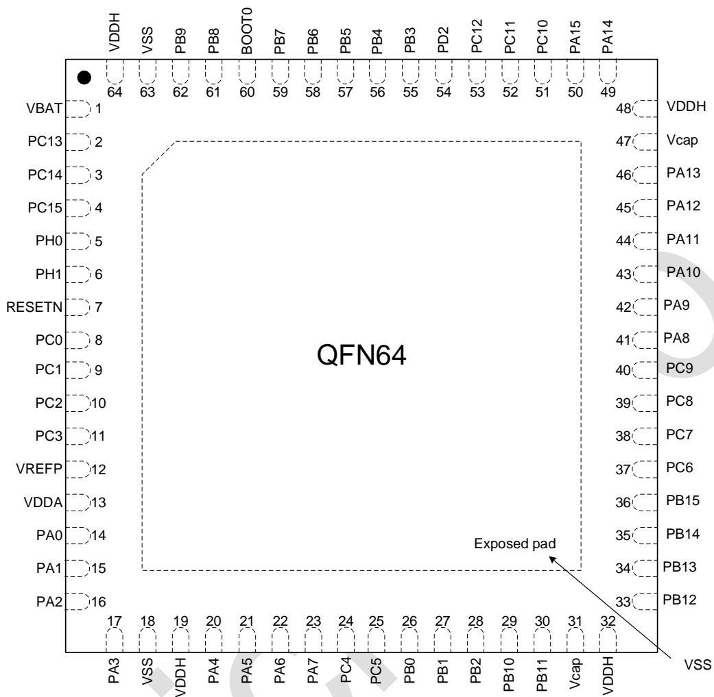
图 3-4: QFN64 引脚分布图
