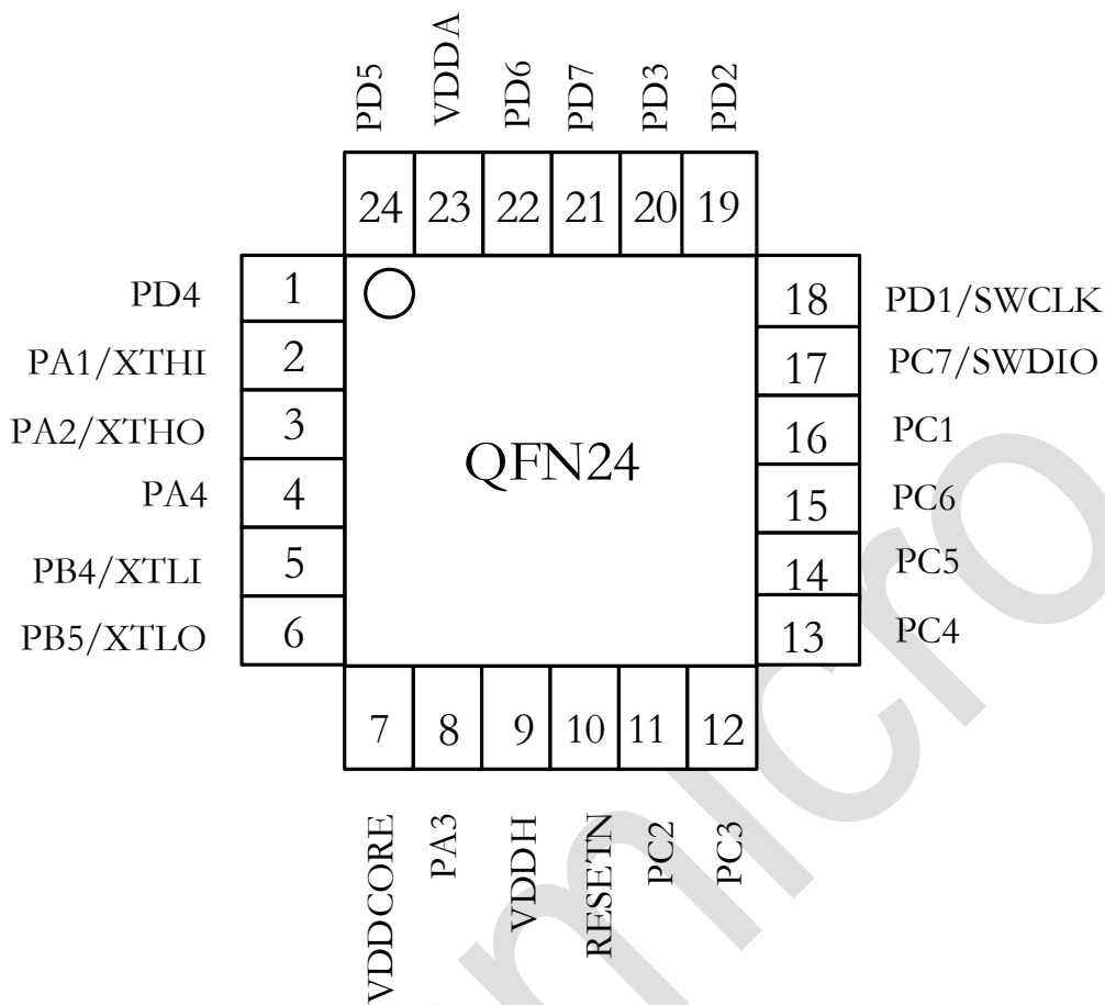
图 3-2: QFN24 管脚分布图
