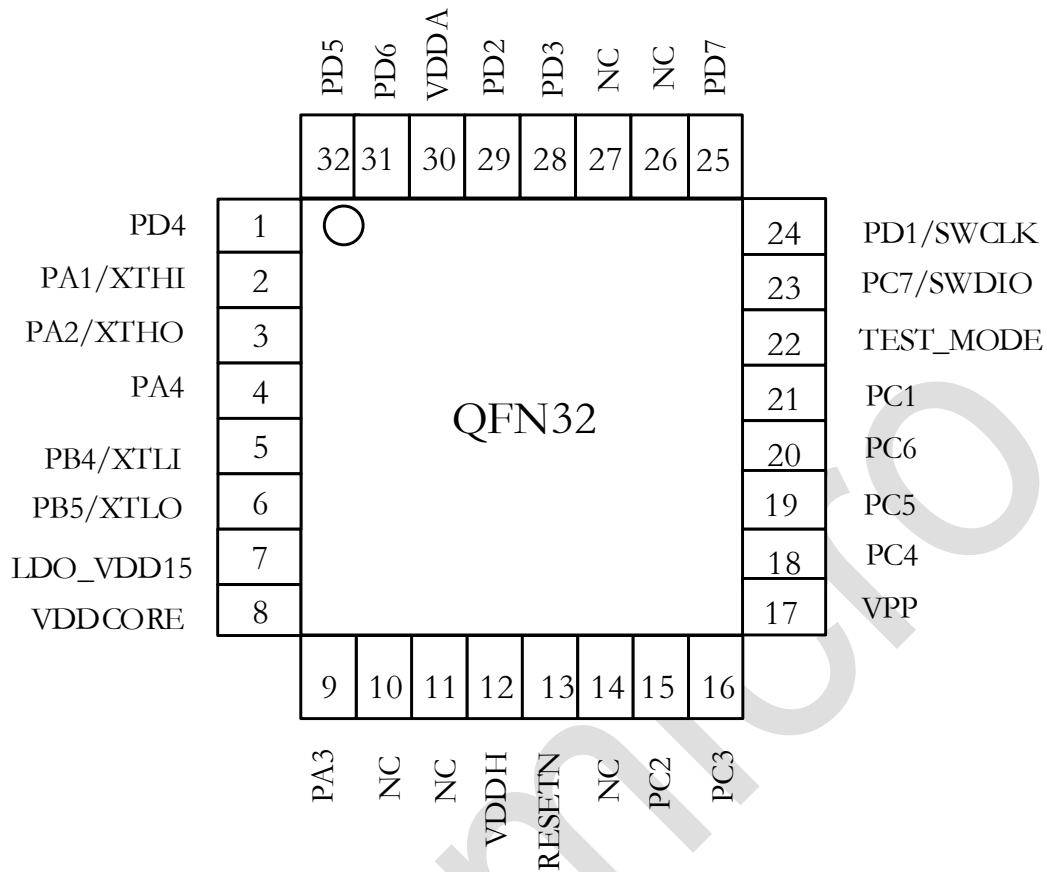
图 3-3: QFN32 管脚分布图（仅用于 EVB 开发板）
