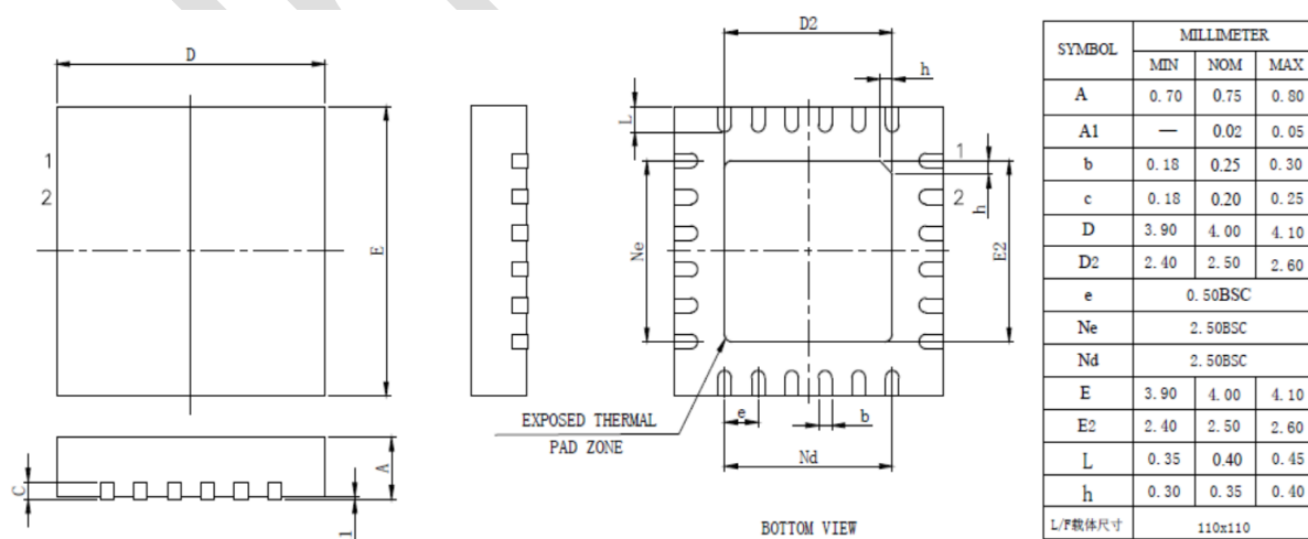
图 5-2: QFN24 封装图
