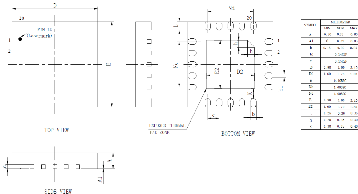
图 5-1: QFN20 封装图
