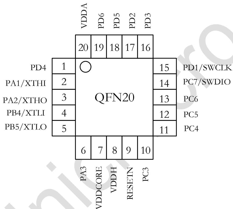
图 3-1: QFN20 管脚分布图
