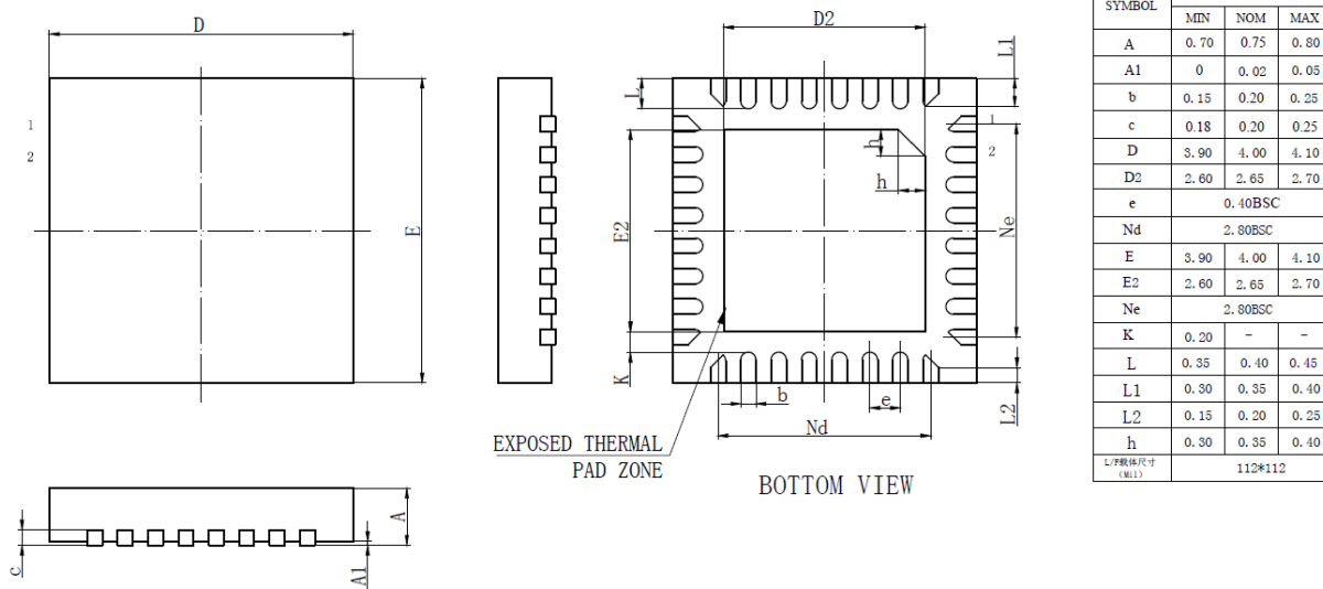
图 5-3: QFN32 封装图
