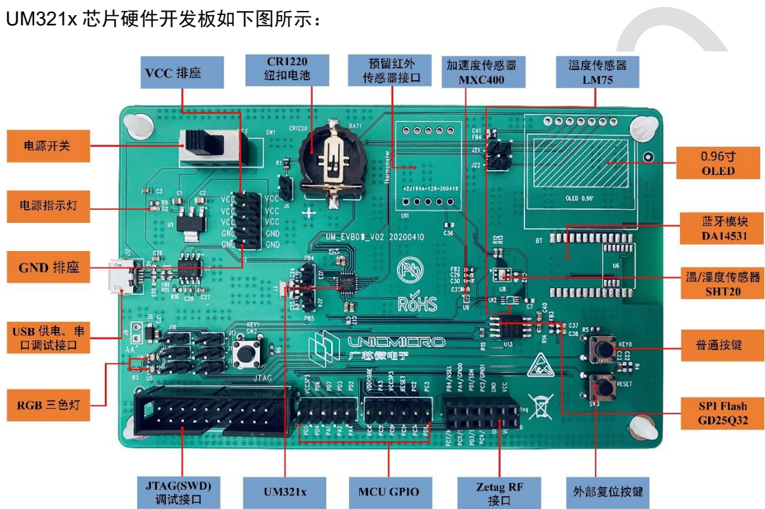
图 2-1: UM321x 芯片硬件开发板图
