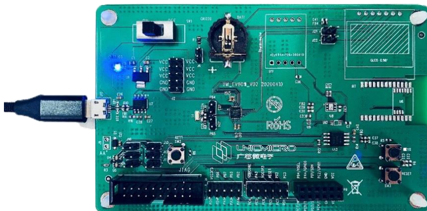
图 2-22：量产环境硬件示意图
