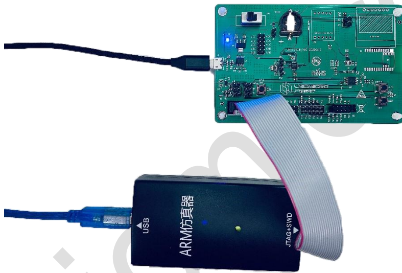
图 2-2: JTAG 仿真调试接线示意图
