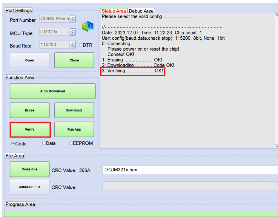
图 2-30: Verify 界面
