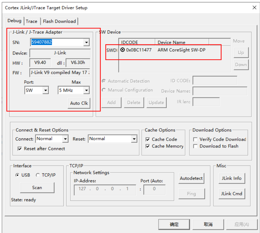
图 2-5: Debug 配置
