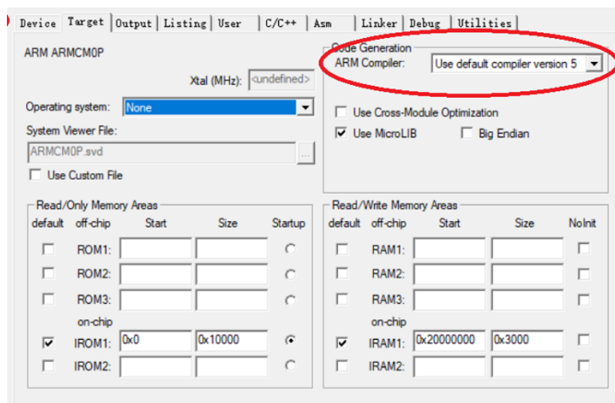
图 2-3: 版本选择
