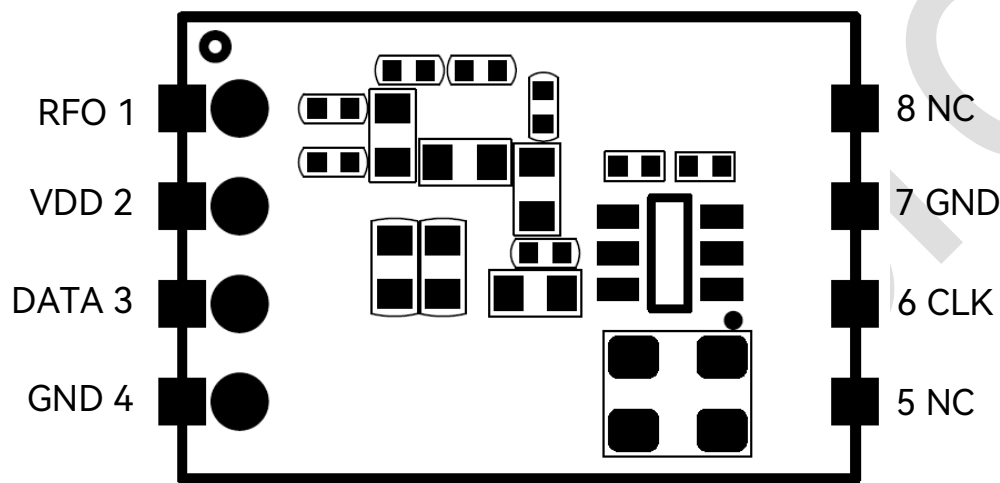
图 2-1：引脚分布图
