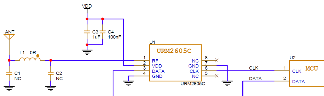
图 4-1: 应用参考图
