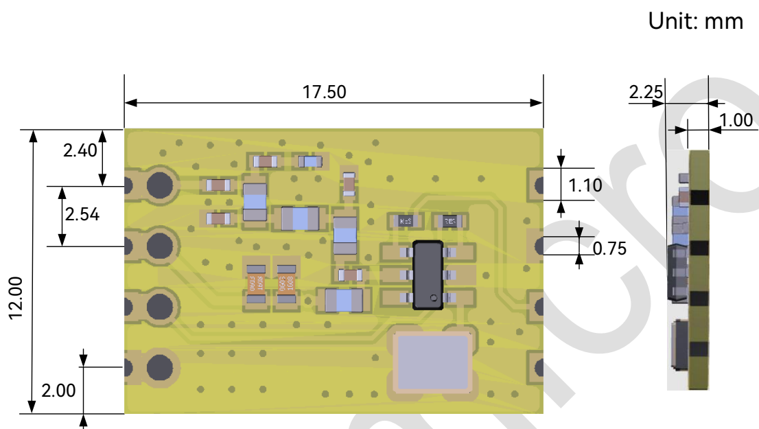
图 5-1: 模块尺寸图
