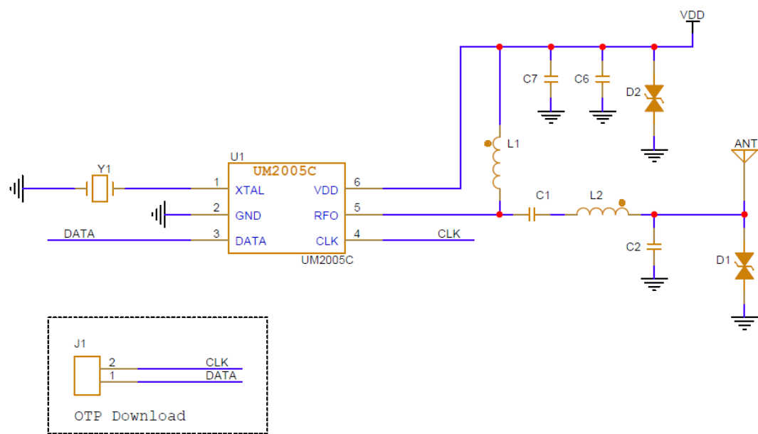
图 8-1：低成本应用参考原理图
