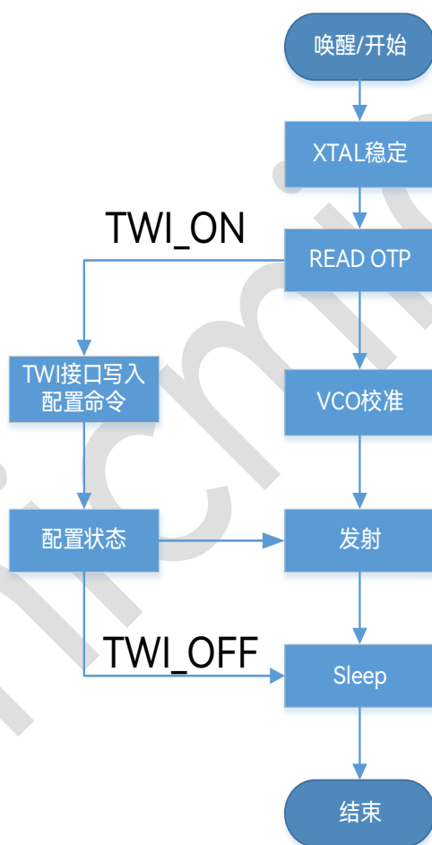
图 6-7：芯片运行状态图
