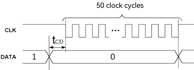
图 6-4：TWI_RST 时序图
