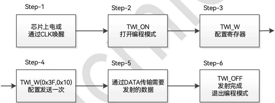
图 7-1：在线配置流程图
