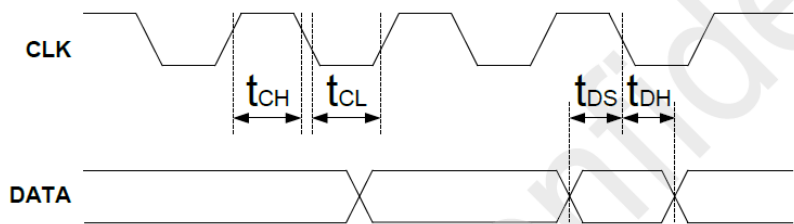
图 6-2: CLK / DATA 时序图
