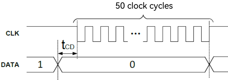
图 6-3：TWI_ON 时序图
