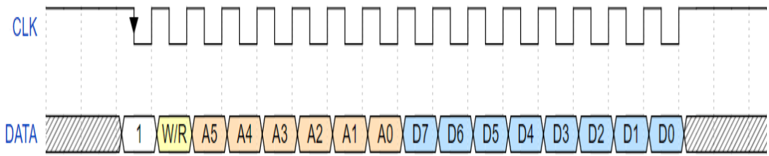
图 6-1: TWI 接口时序图
