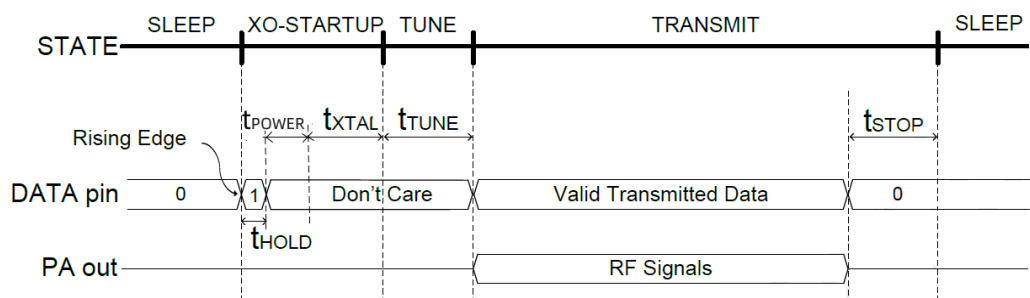
图 7-3：数据直通时序图
