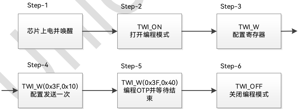
图 5-2：配置 OTP 流程
