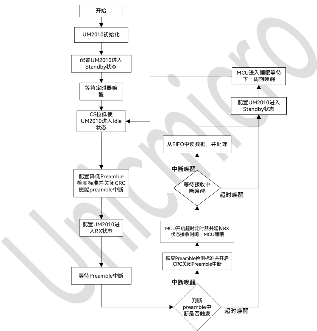
图 3-6：接收检测 Preamble 中断（Standby 模式）流程图
