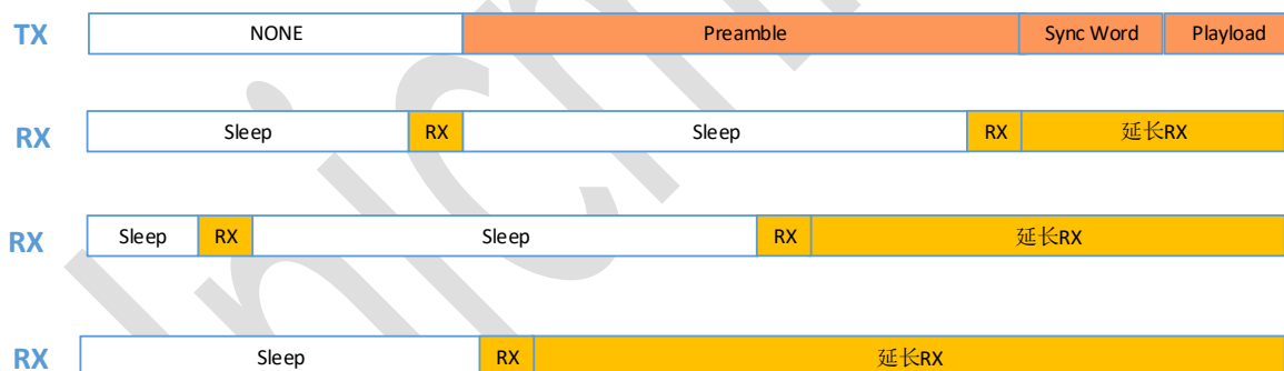
图 2-2: Preamble 中断检测低功耗通信时序图
