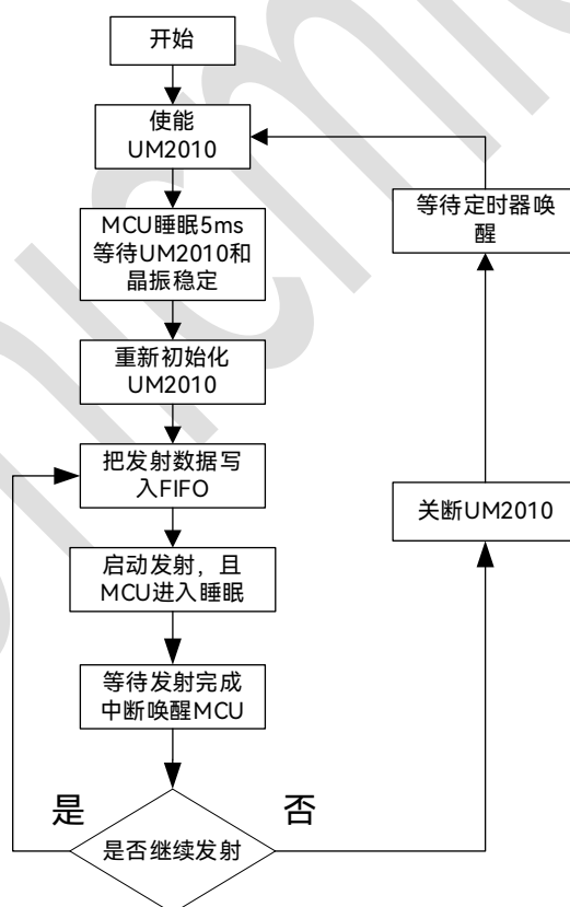
图 3-1：低功耗发射（Shutdown 模式）流程图
