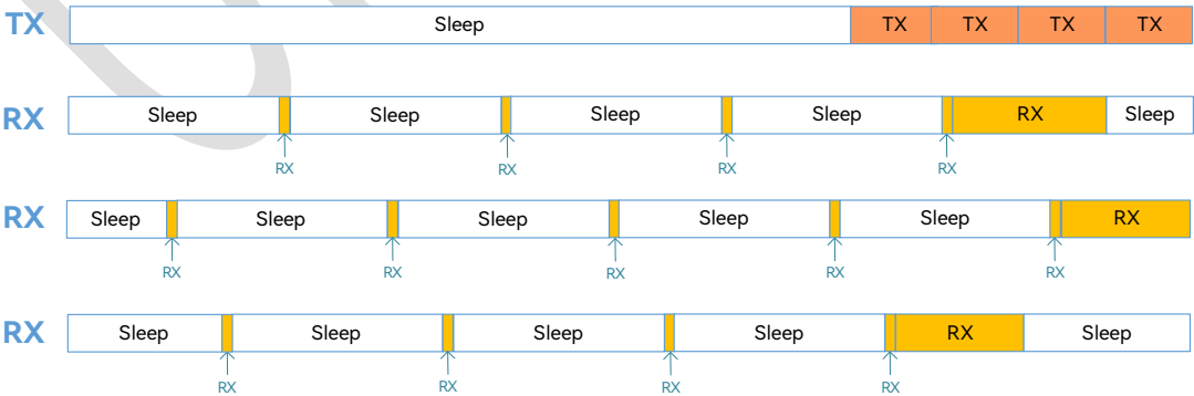
图 2-1：RSSI 检测低功耗通信时序图
