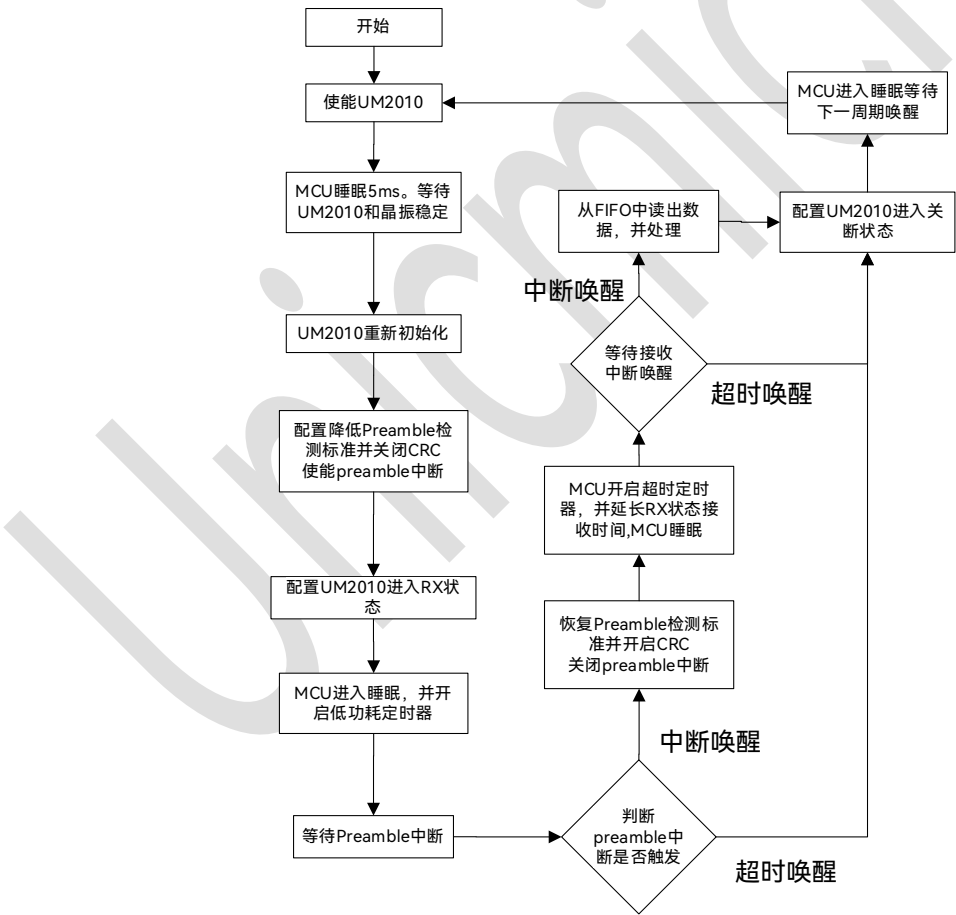
图 3-4：接收检测 Preamble 中断（Shutdown 模式）流程图
