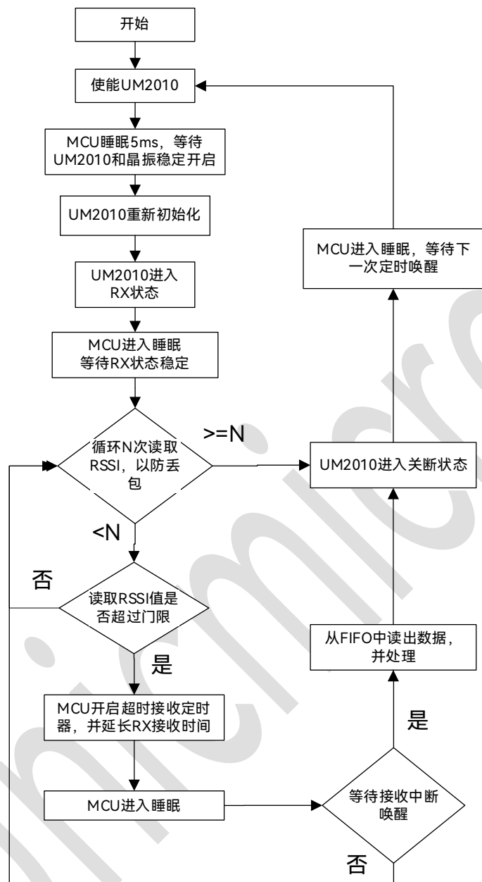
图 3-3：接收检测 RSSI（Shutdown 模式）流程图
