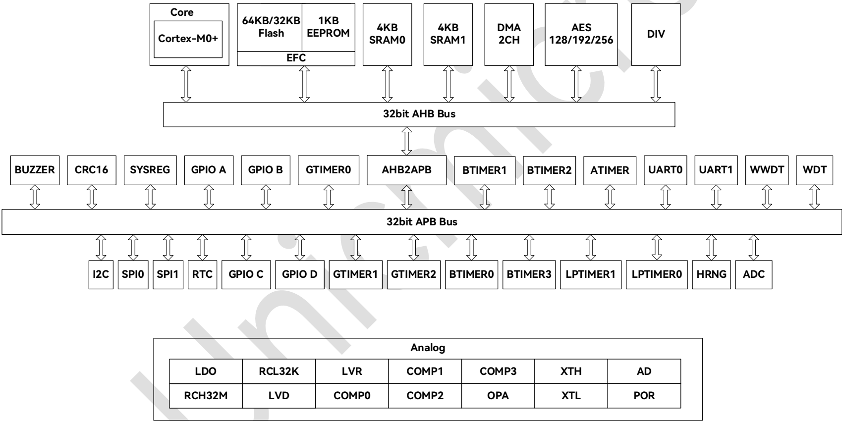
图 1-1：功能框图
