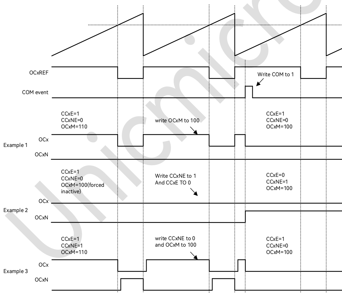
图 16-11: 产生六步 PWM, 使用 COM 的例子(OSSR=1)
