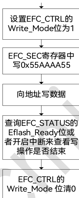
图 6-1：写操作流程
