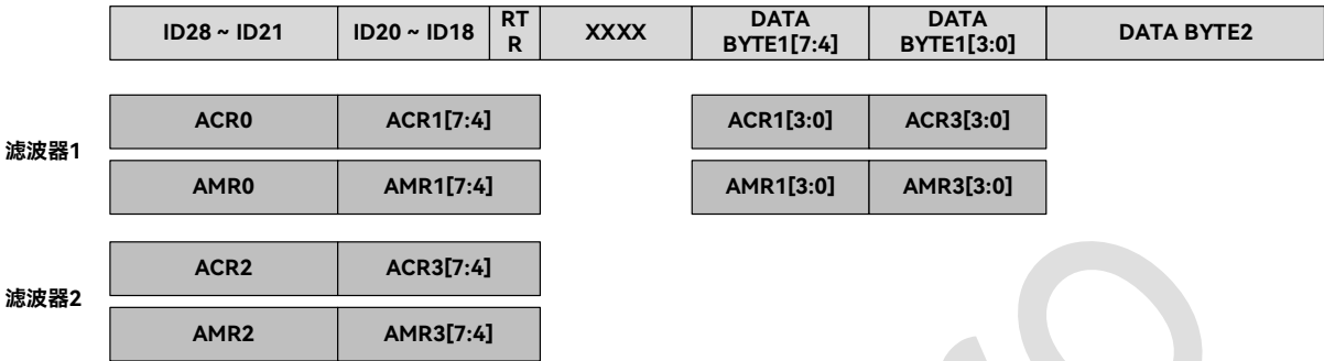
图 14-6：标准帧双滤波器模式
