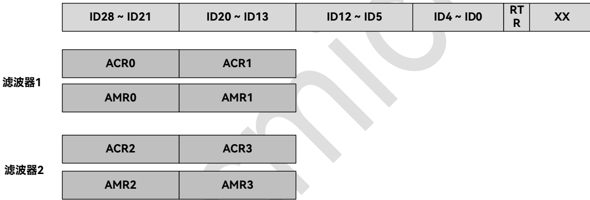
图 14-7：扩展帧双滤波器模式
