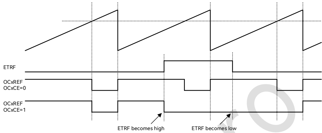
图 16-12: ETR 信号清除 ATIMER 的 OCxREF
