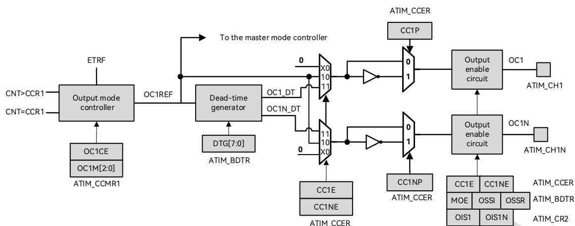
图 16-4: 捕获/比较通道的输出部分(通道 1 至 3)
