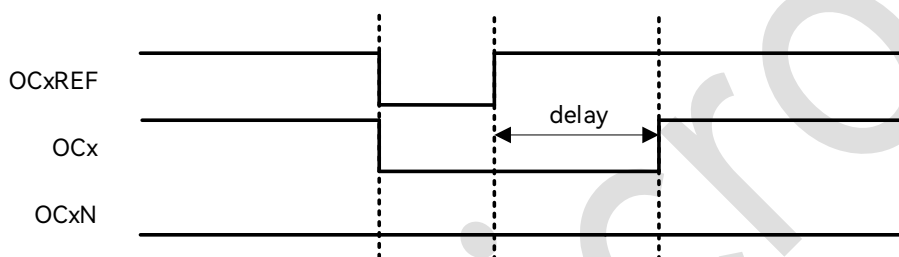
图 16-8: 死区波形延迟大于负脉冲
