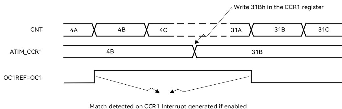
图 16-6：输出比较模式，翻转 OC1
