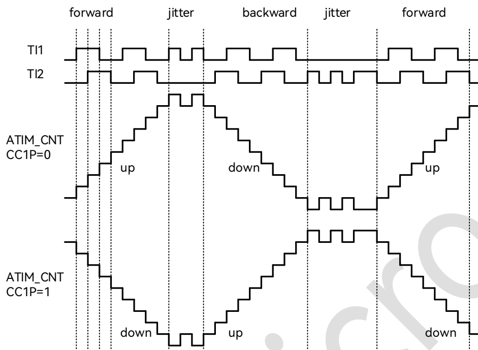
图 16-13: 编码器模式下的计数器操作实例
