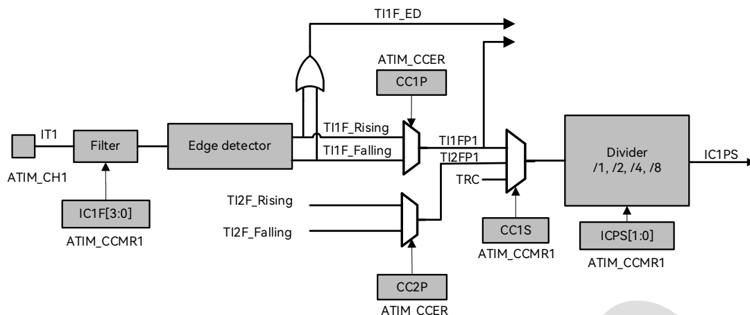
图 16-2: 捕获/比较通道(通道 1 输入部分)
