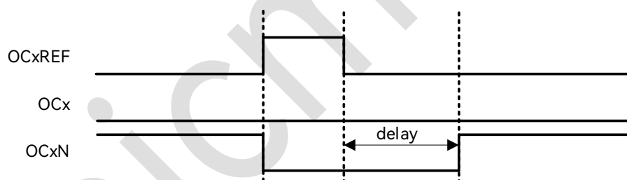
图 16-9: 死区波形延迟大于正脉冲
