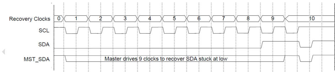
图 26-1: 使用 9 个 SCL 时钟恢复 SDA 图
