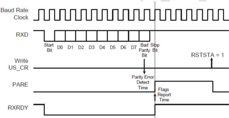
图 30-17：检验错误时序图
