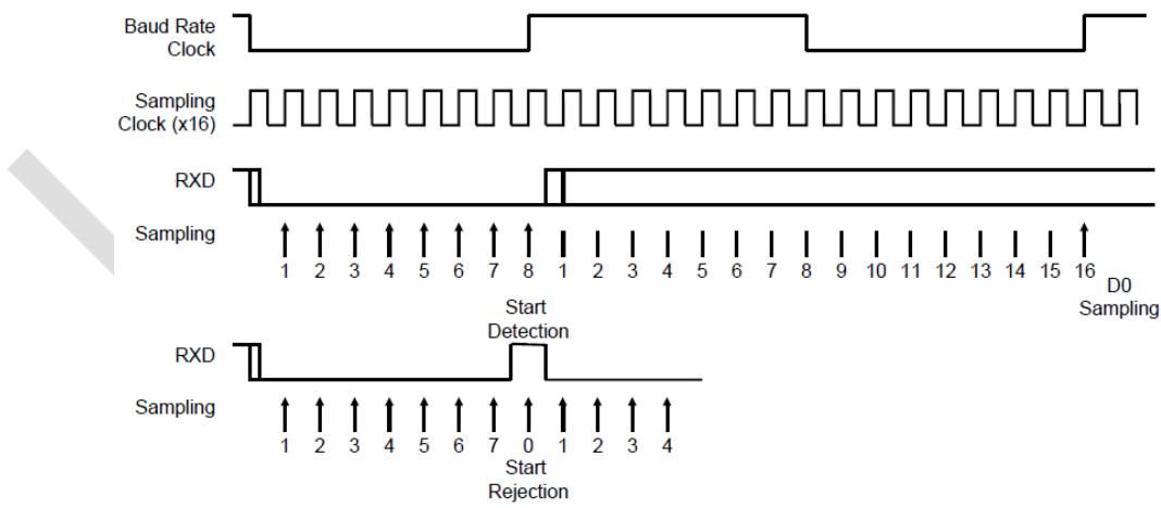
图 30-7：异步起始位检测
