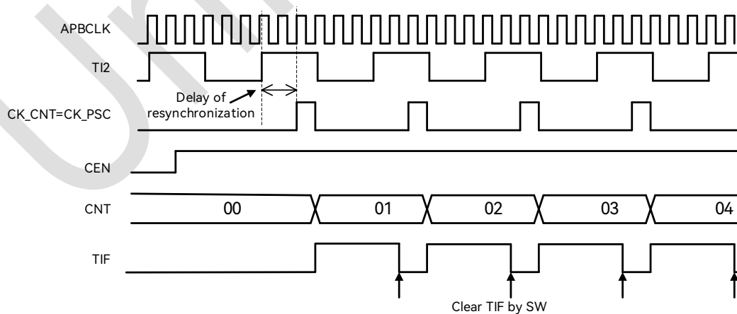
图 18-19：外部时钟模式 1 下的时序图
