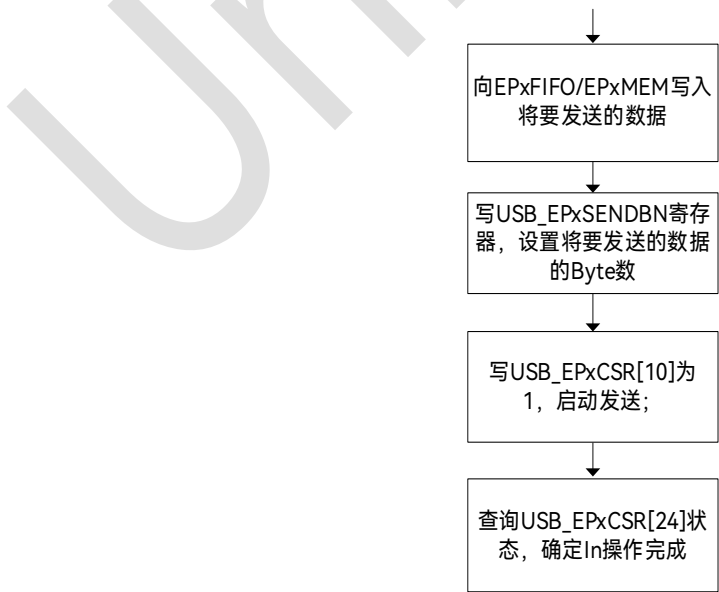
图 35-2: USB Endpoint In 传输流程图
