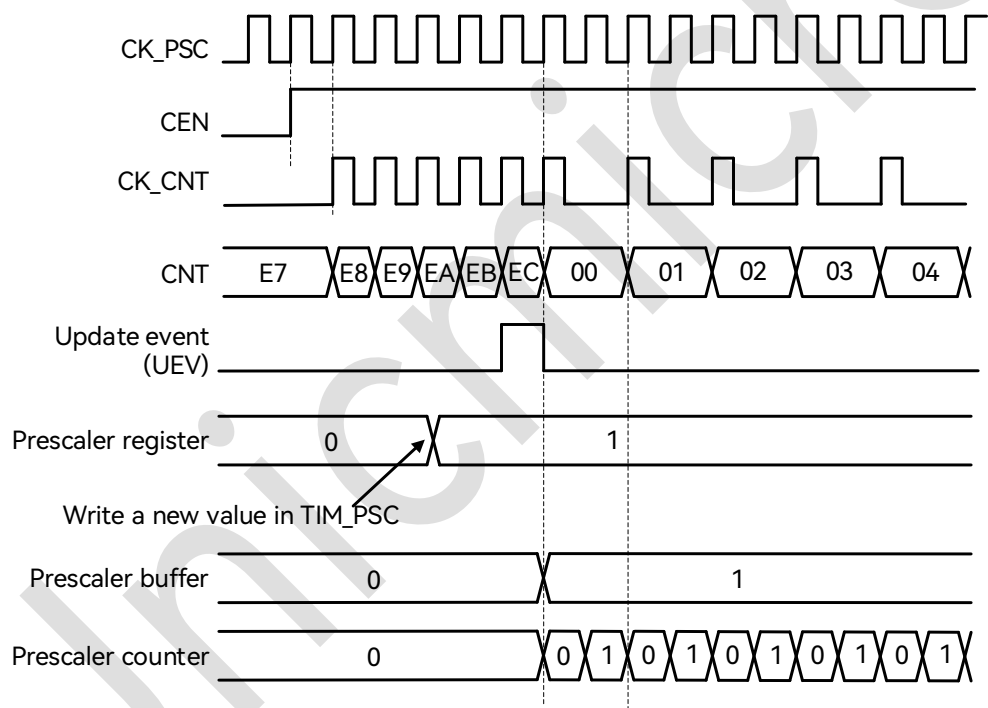
图 20-1: 预分频从 1 变为 2 的波形
