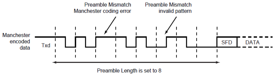
图 30-10：前同步信号模式不匹配
