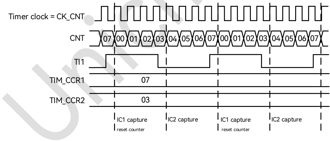
图 19-26: PWM 输入捕获模式时序
