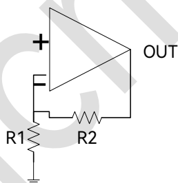
图 39-1 外部放大电路连接图
