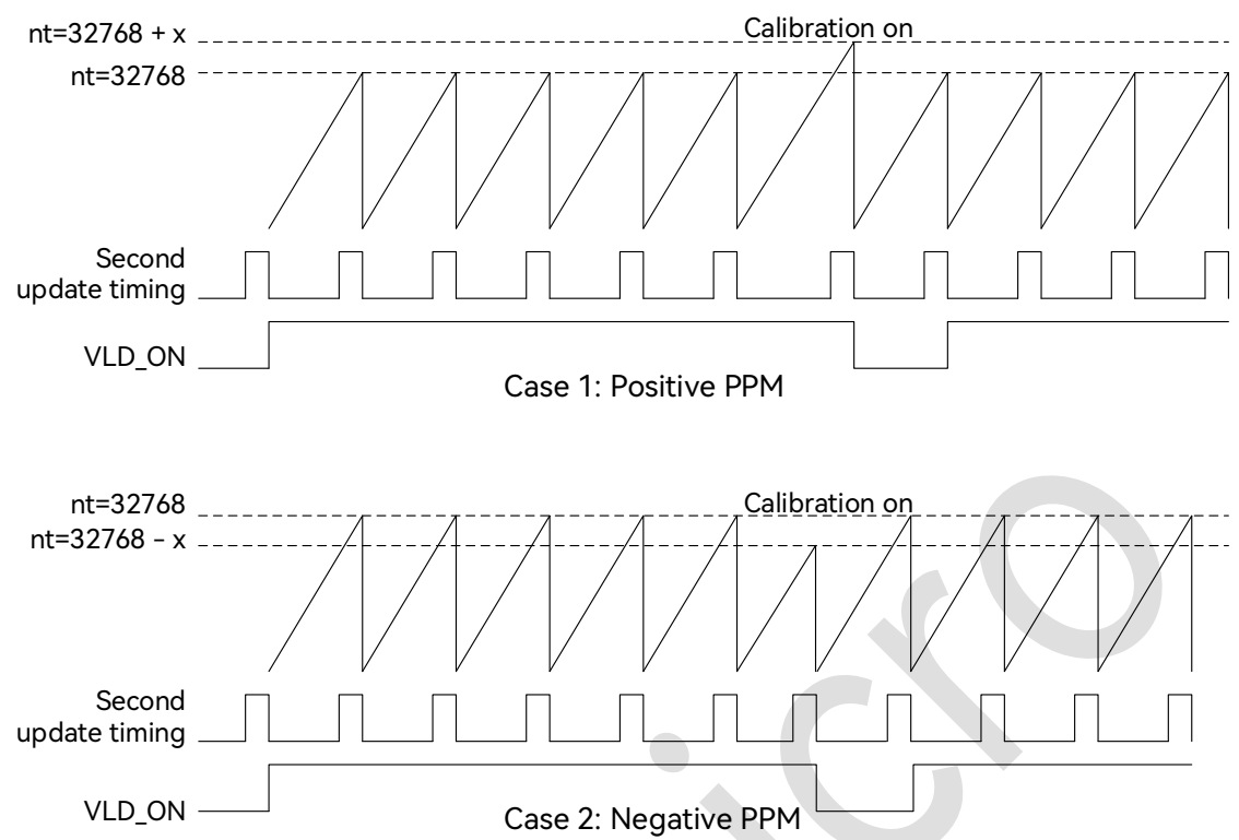
图 24-2：震荡校准
