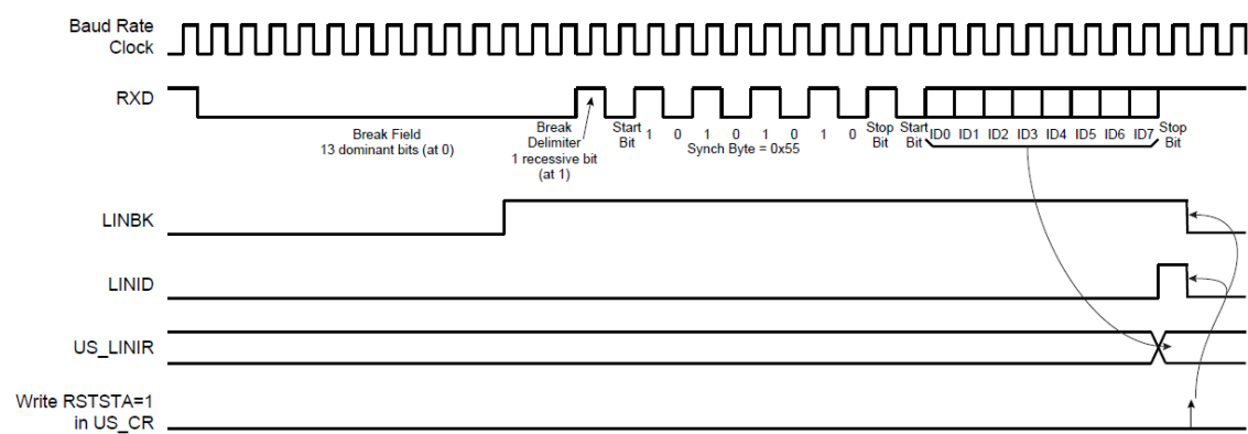
图 30-30：报文接收
