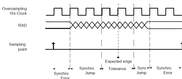
图 30-6: 位同步图
