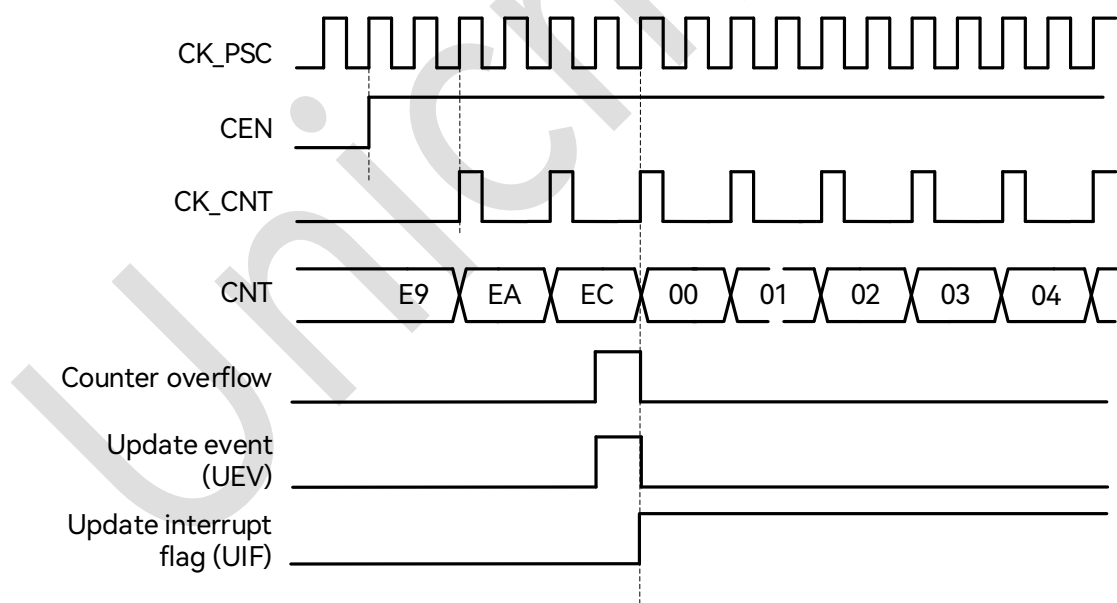
图 20-4: 向上计数波形，内部时钟 2 分频
