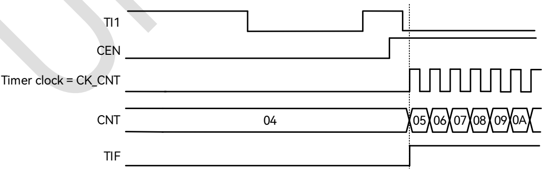
图 19-35: 触发器模式下的时序
