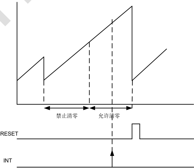
图 23-1：WWDT 计数器刷新时序图
