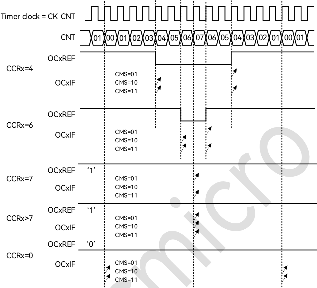
图 18-30：中央对齐的 PWM 波形（ARR=7）图
