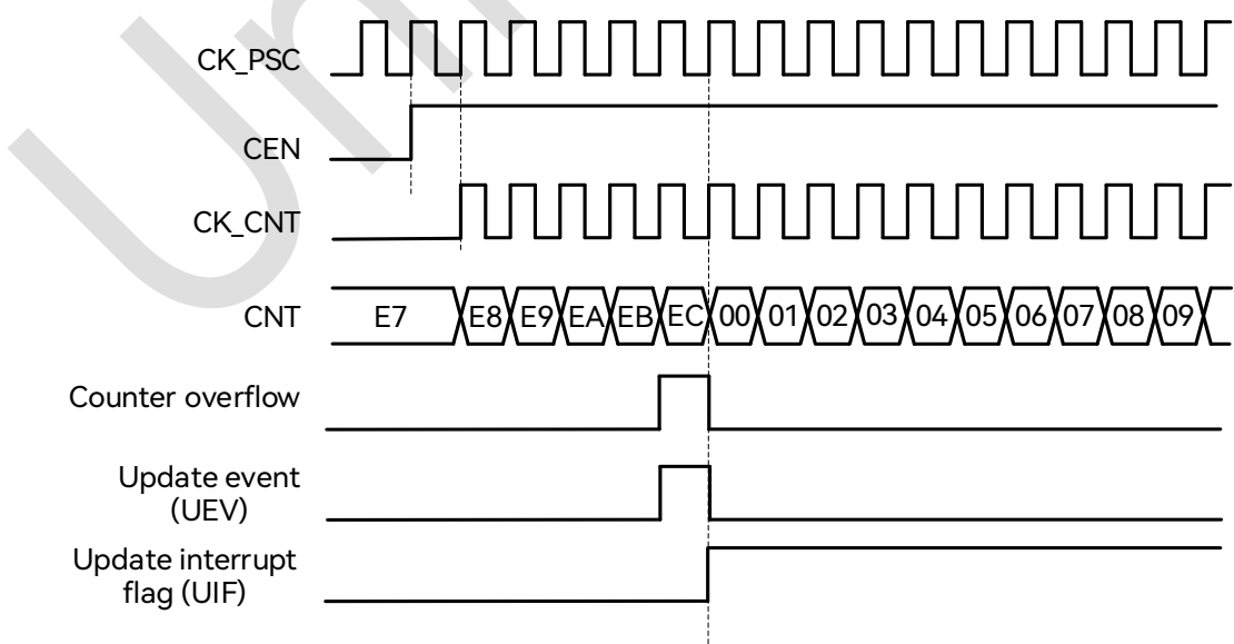
图 19-4: 向上计数波形，内部时钟不分频
