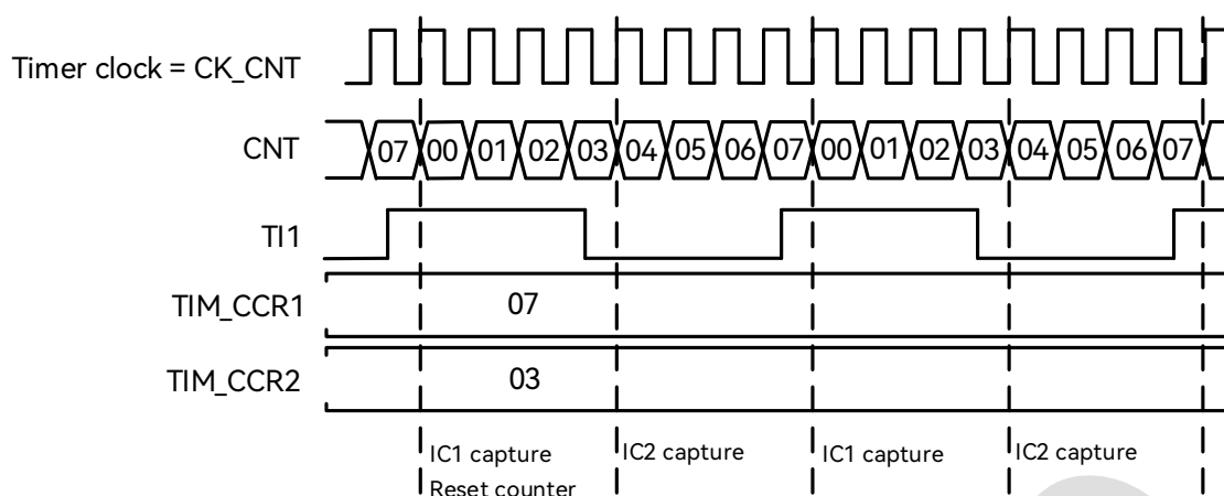
图 18-27: PWM 输入捕获模式时序图
