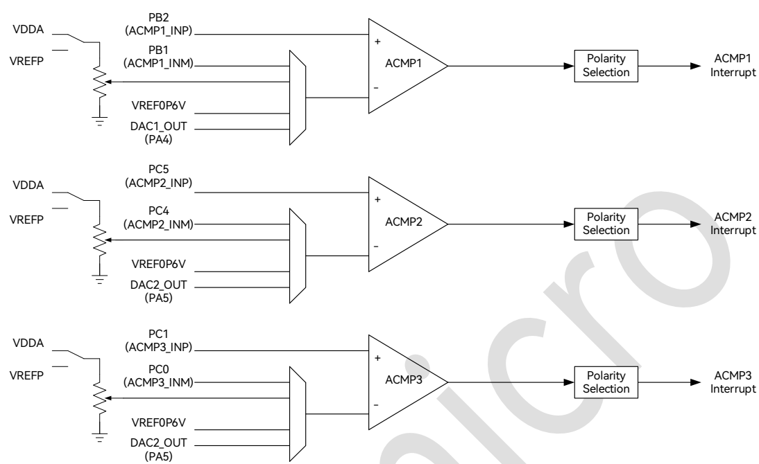
图 38-1: ACMP 系统框图
