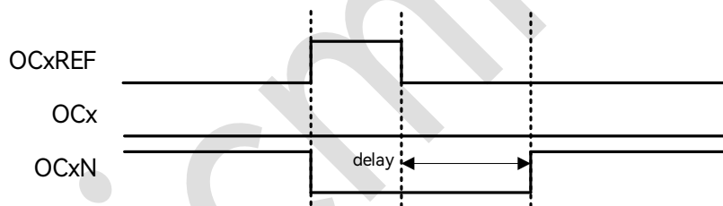
图 18-33: 死区波形延迟大于正脉冲时序图
