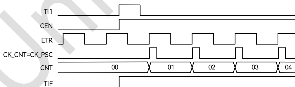
图 19-36：外部时钟模式 2 + 触发模式下的时序
