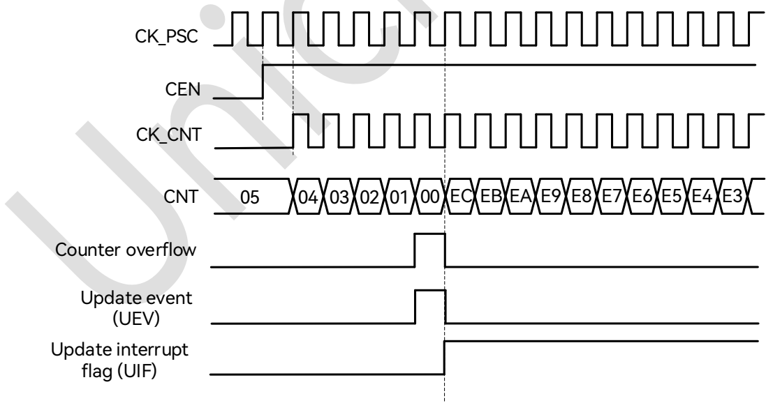
图 18-8：向下计数，内部时钟不分频图
