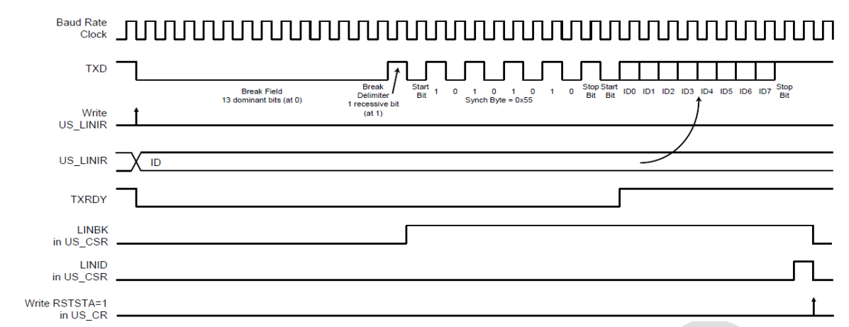
图 30-29：报文传输
