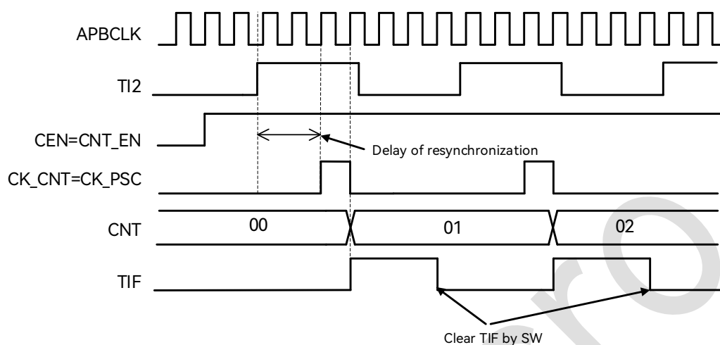
图 19-17: 外部时钟模式 1 下的时序
