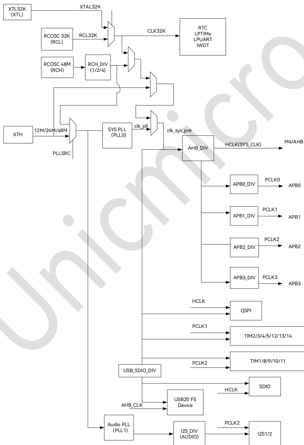
图 6-1: 时钟单元
