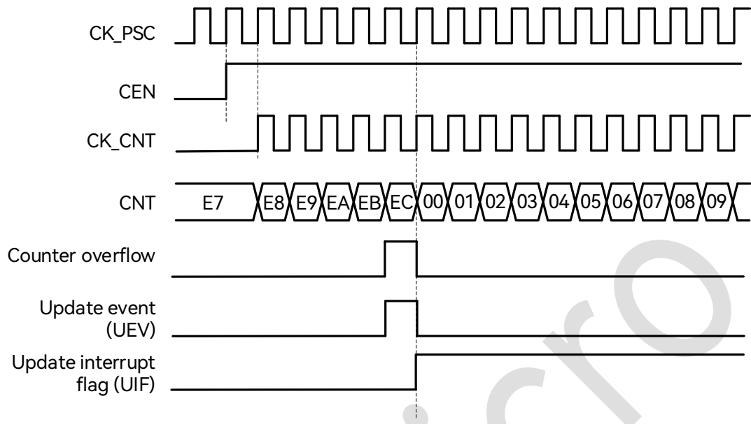
图 20-3: 向上计数波形，内部时钟不分频
