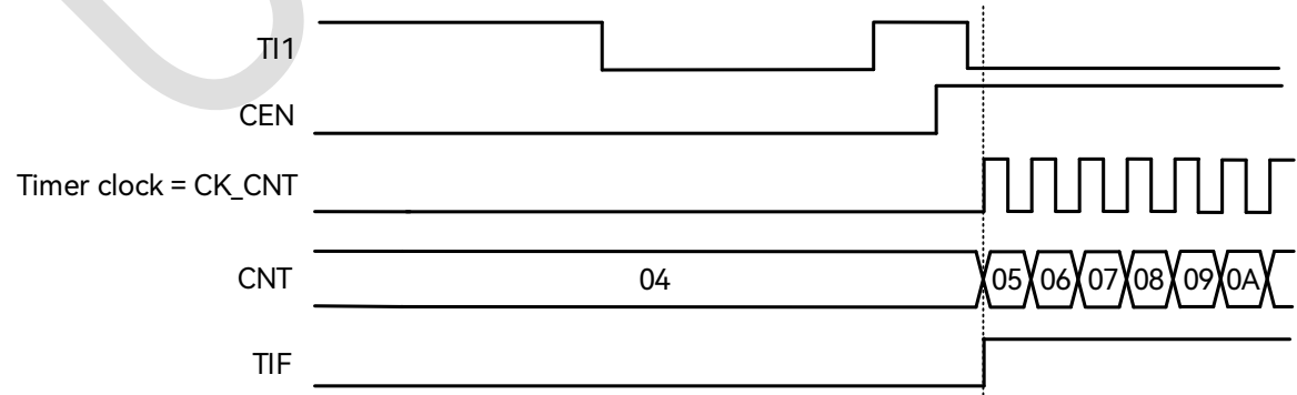
图 18-41：触发器模式下的时序图
