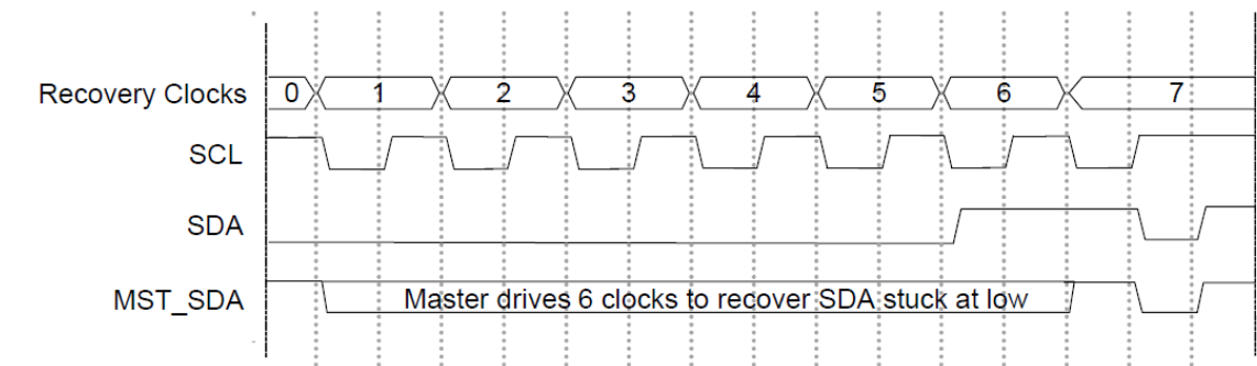
图 26-2: 使用 6 个 SCL 时钟恢复 SDA 图
