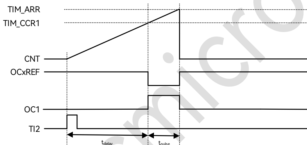
图 19-30：单脉冲模式的例子
