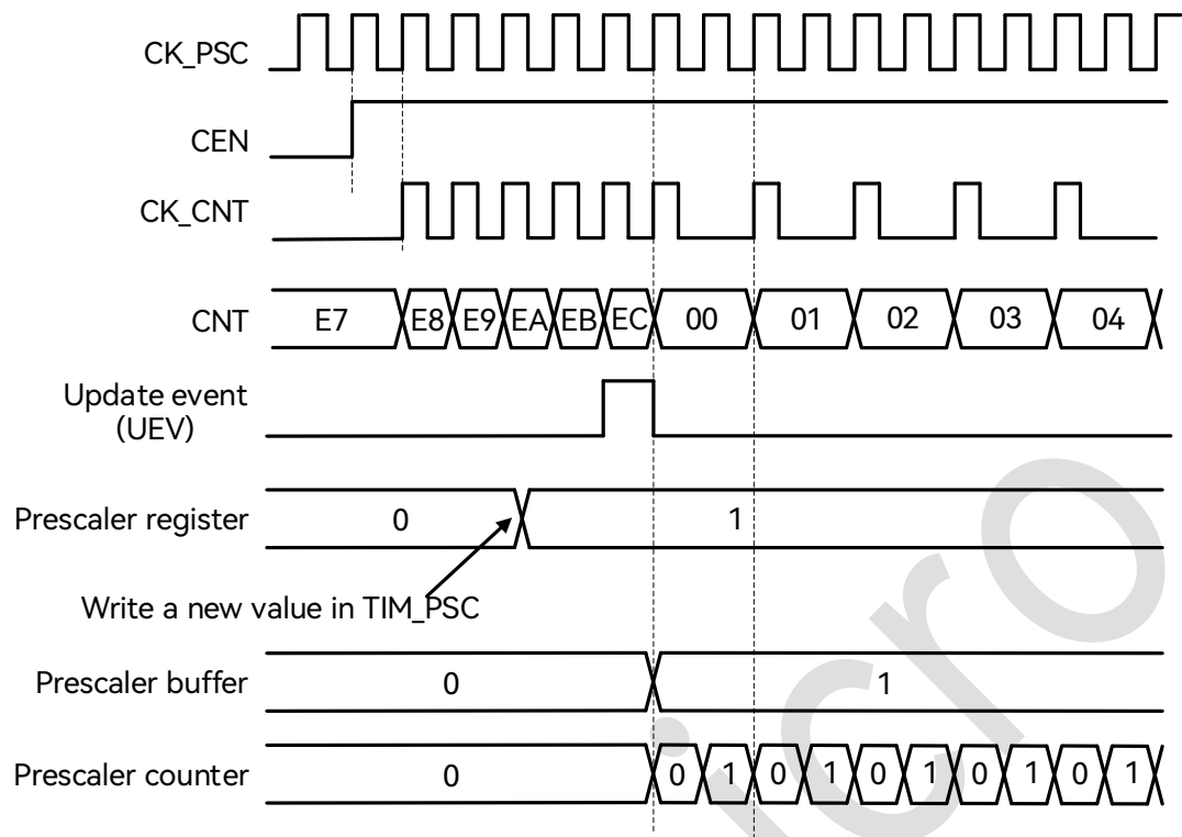
图 18-2: 预分频从 1 变为 2 的波形图
