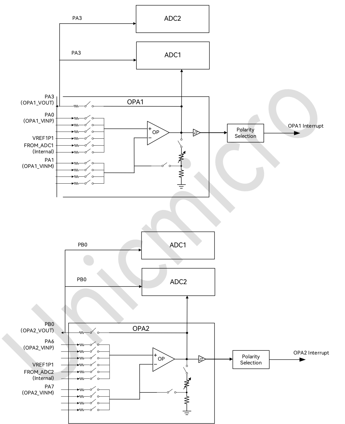
图 39-1: OPA 系统框图
