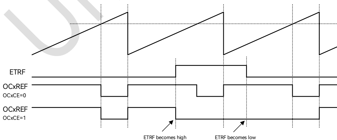
图 18-37: ETR 信号清除 TIM 的 OCxREF 时序图
