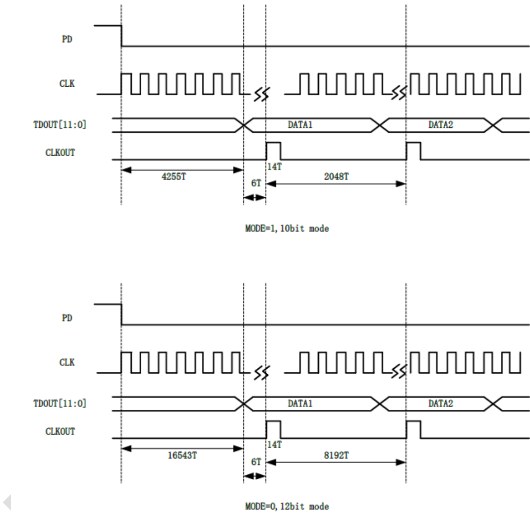
图 40-1：温度传感器转换时序图
