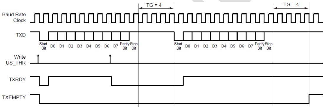
图 30-18：时间保护操作时序图
