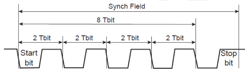
图 30-31：同步域
