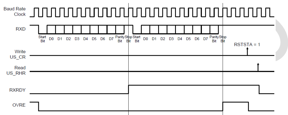
图 30-16: 接收器状态
