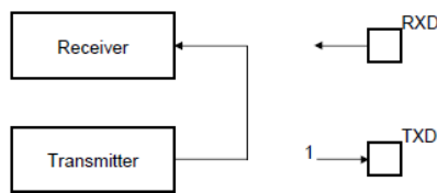
图 30-46: USART 本地环回模式
