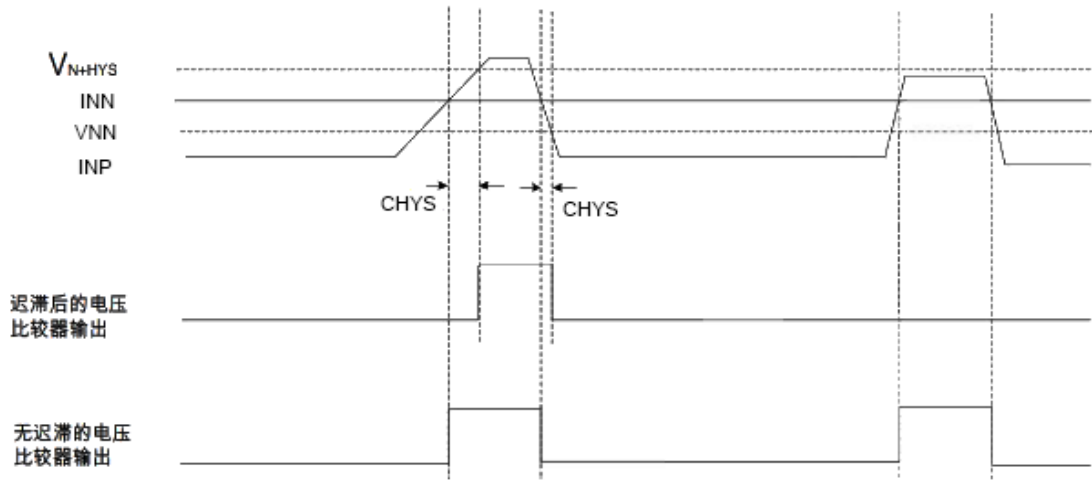
图 38-3：带迟滞功能的电压比较功能图
