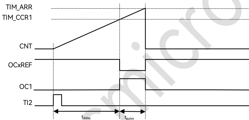
图 18-36: 单脉冲模式时序图
