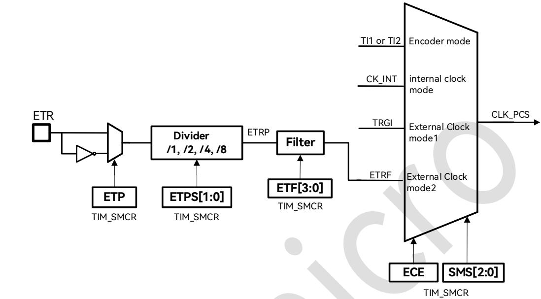
图 18-20：外部触发输入框图
