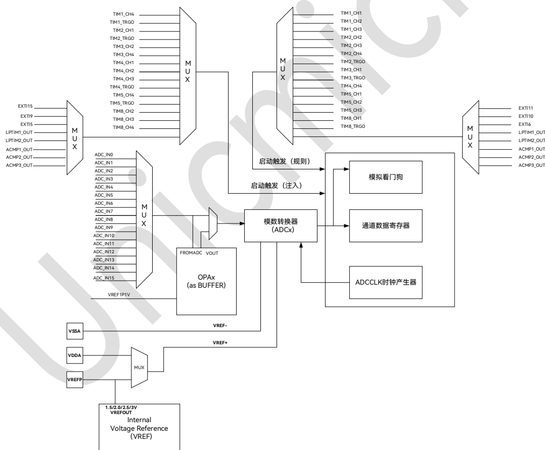
图 36-1: ADC 系统框图
