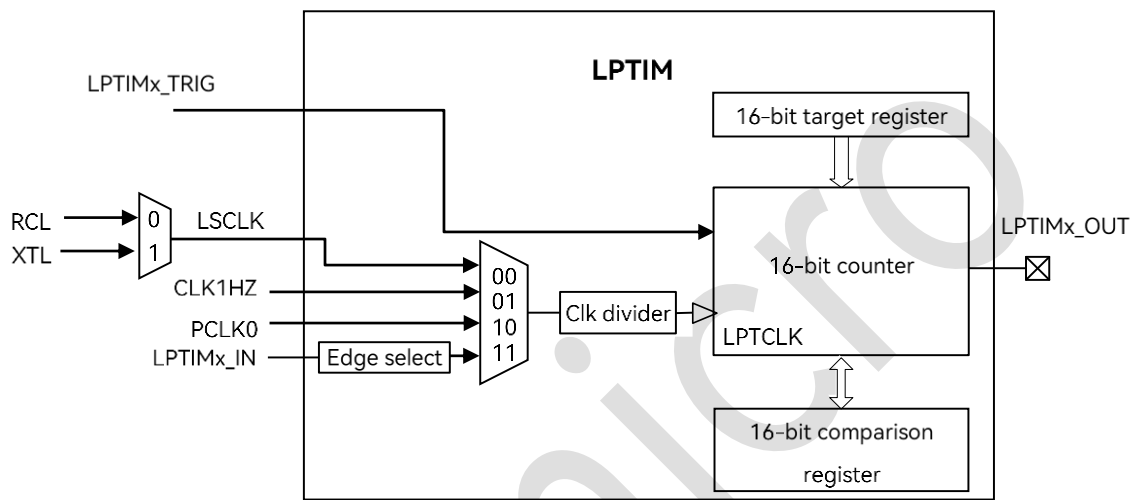
图 21-1: 系统框图
