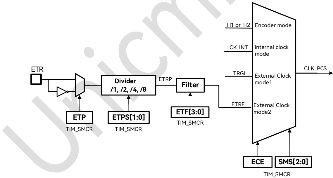
图 19-19：外部触发输入框图
