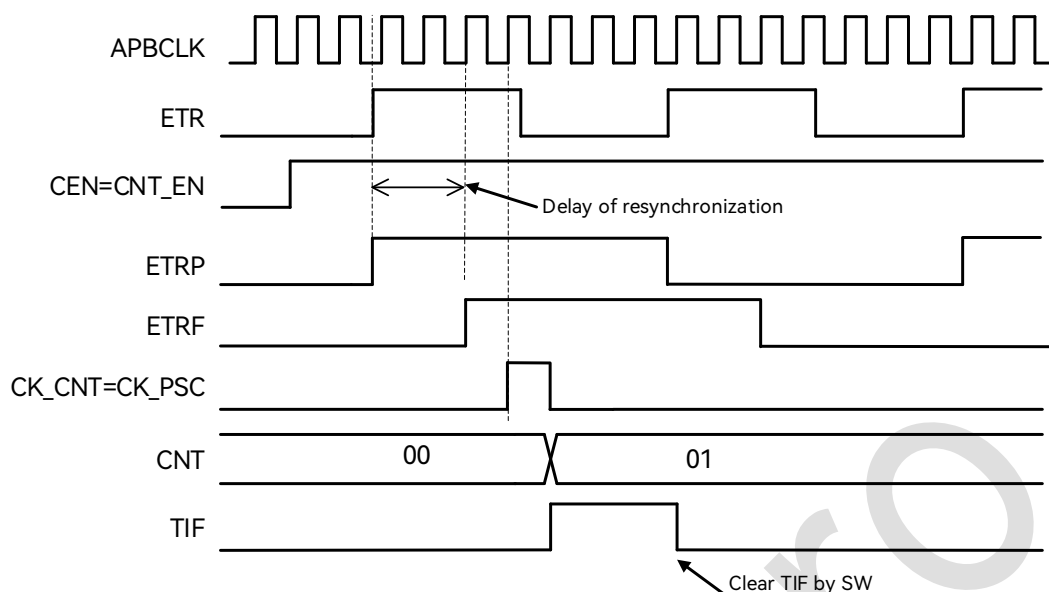
图 19-20: 外部时钟模式 2 下的时序 1
