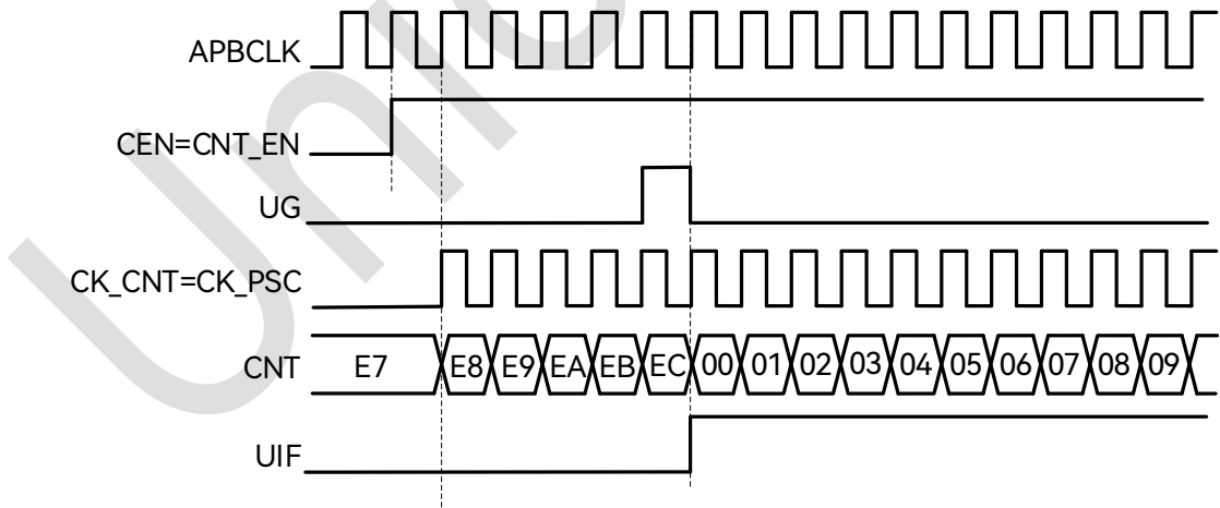
图 18-16：内部时钟源模式，时钟分频因子为 1 时序图
