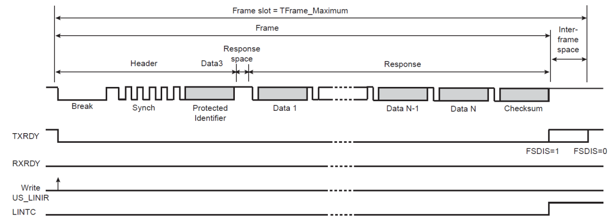
图 30-37: 主节点配置, NACT = IGNORE
