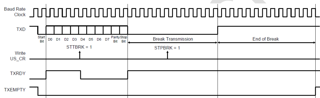
图 30-20：中断的传输
