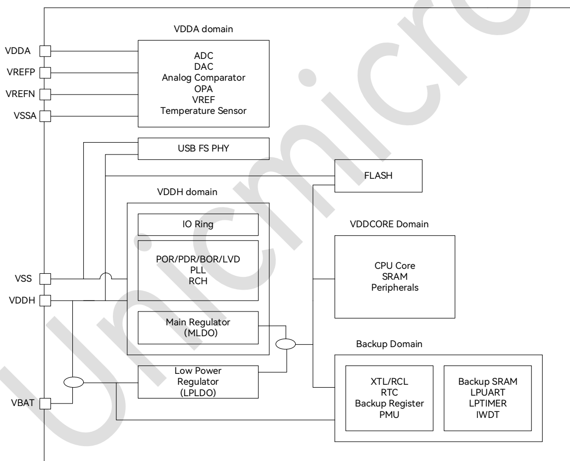
图 5-1：系统供电方案框图
