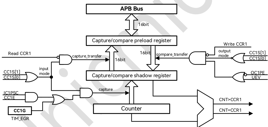
图 19-23: 捕获/比较通道 1 的主电路
