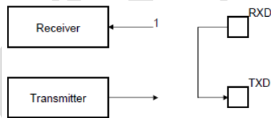
图 30-47: USART 远程环回模式
