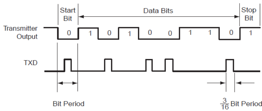
图 30-25: IrDA 调制
