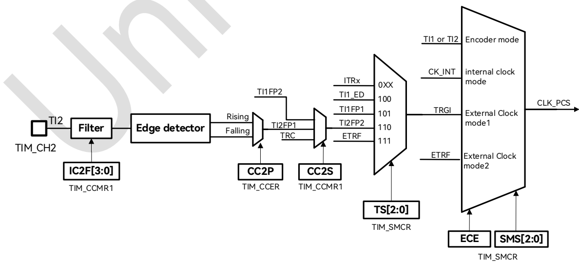
图 19-16：外部时钟连接例子
