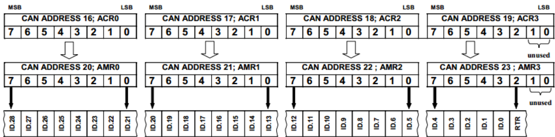
图 25-4：单过滤器扩展帧对应位格式
