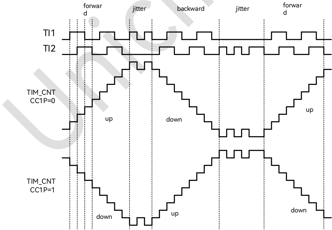
图 19-32: 编码器模式下的计数器操作实例
