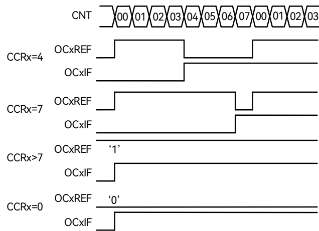
图 19-28: 边沿对齐的 PWM 波形 (ARR=7)
