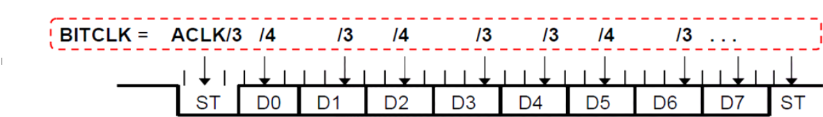
图 29-3：LPUART 接收时序图
