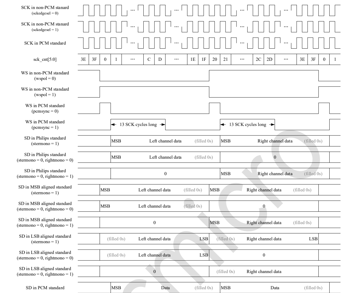
图 27-2: 32 位声道的 I2S 信号波形
