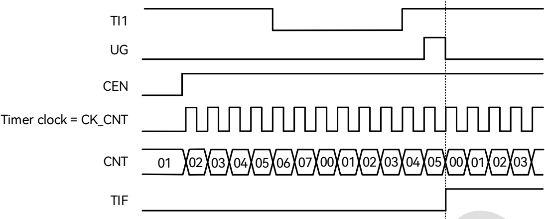
图 19-33: 复位模式下的时序
