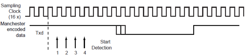
图 30-9：异步起始位检测
