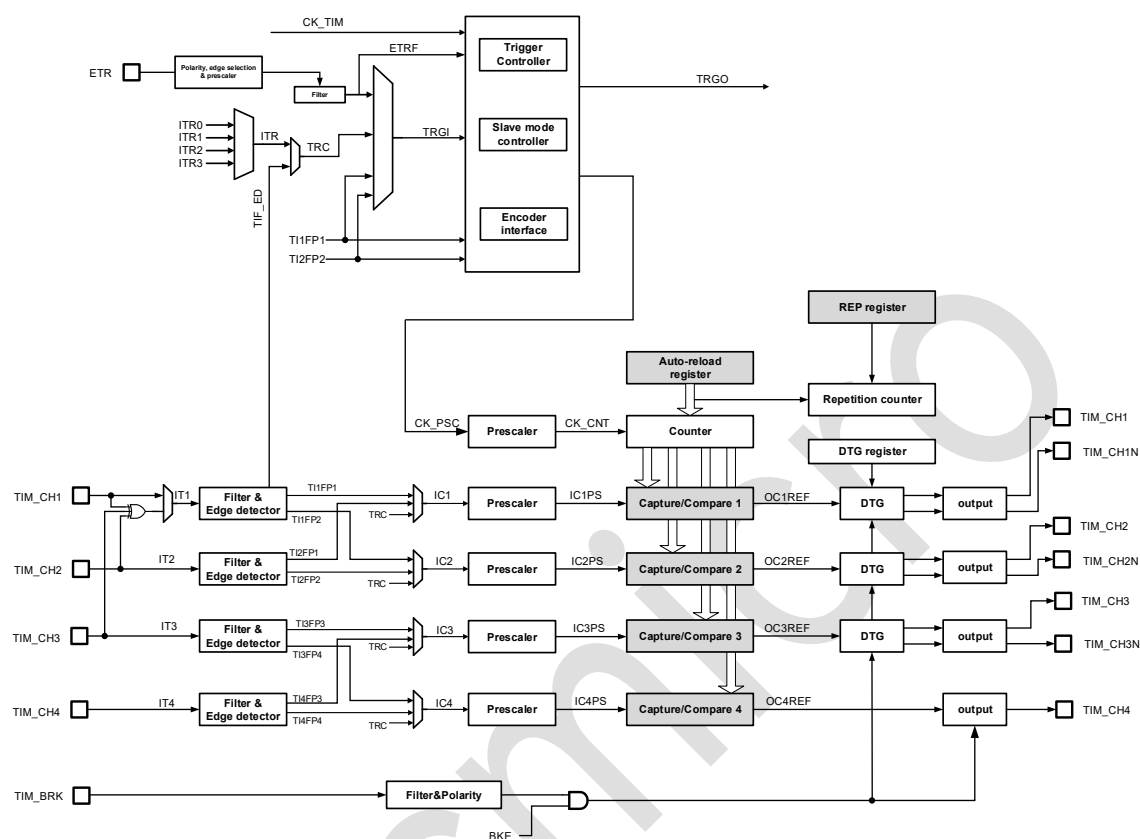
图 18-1: TIM1 & TIM8 系统框图
