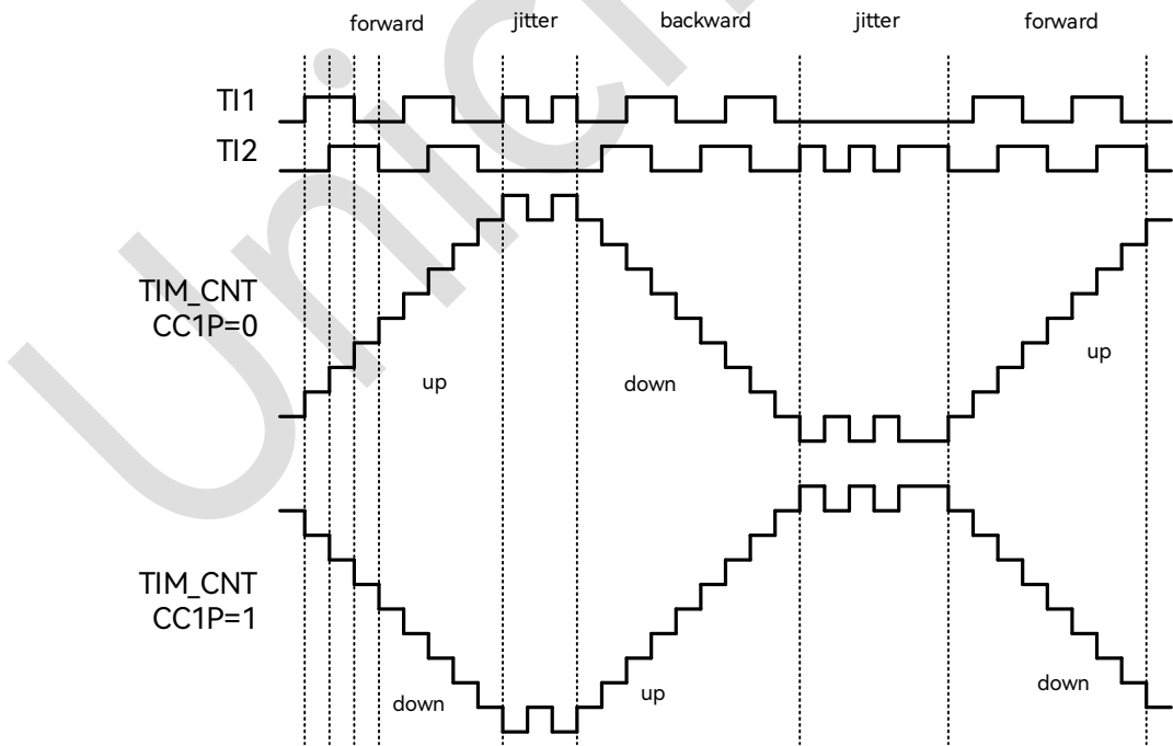
图 18-38: 编码器模式下的计数器操作实例图
