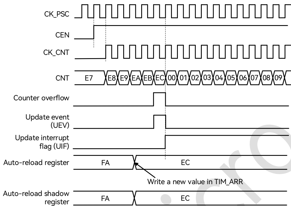
图 20-5: ARPE=0 (TIM_ARR 没有预装载) 时的更新事件
