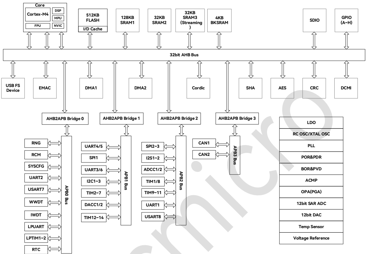
图 3-1: 总线架构图
