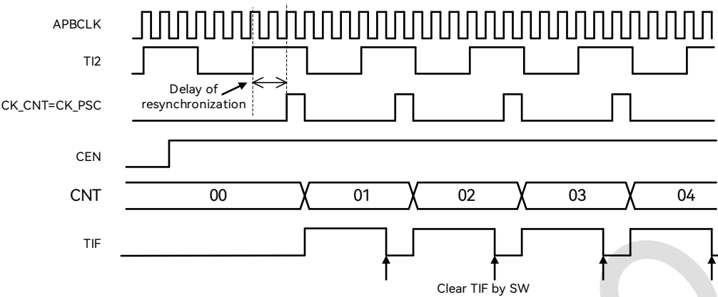
图 19-18：外部时钟模式 1 下的时序
