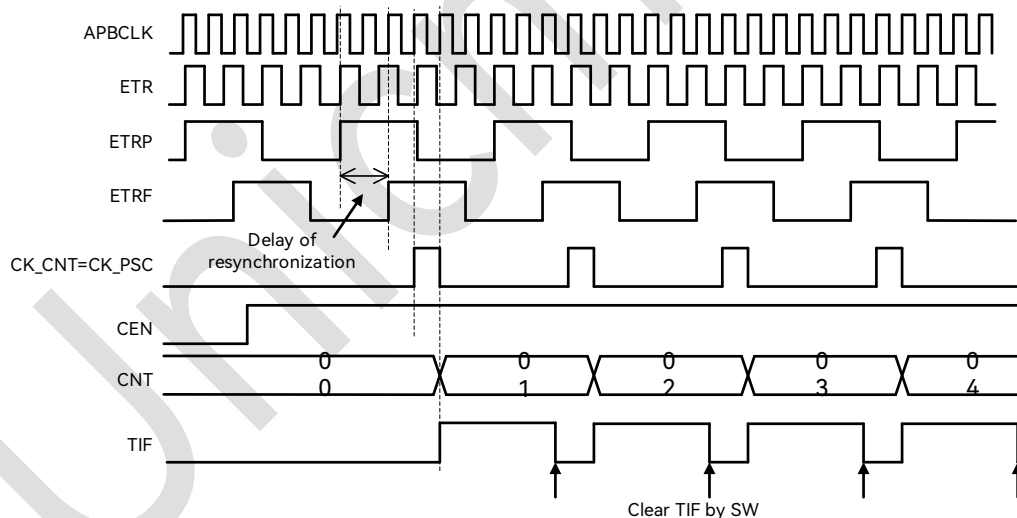
图 18-22: 外部时钟模式 2 下的时序 2 图
