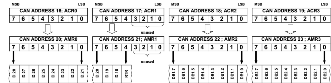
图 25-3：单过滤器标准帧对应位格式
