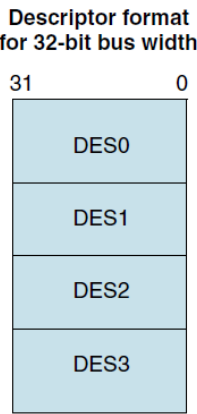
图 33-3：DES0~DES3 结构图
