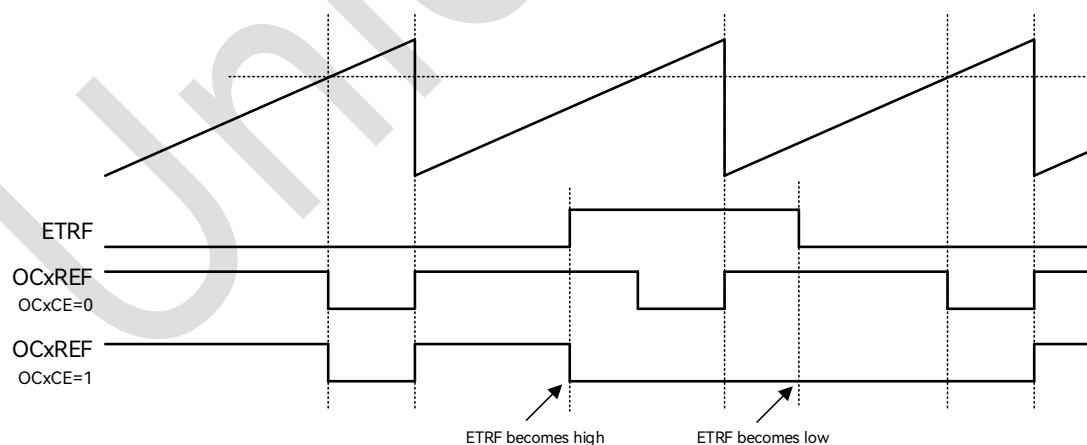
图 19-31: ETR 信号清除 TIM 的 OCxREF
