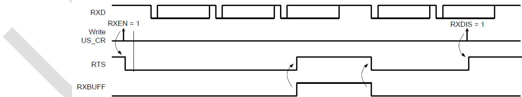
图 30-22：允许硬件握手时接收器工作行为
