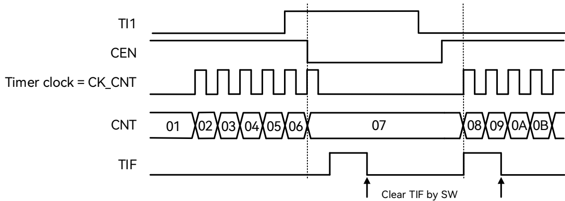
图 18-40：门控模式下的时序图
