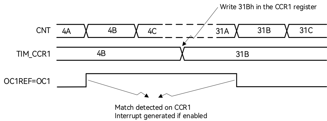
图 19-27：输出比较模式，翻转 OC1
