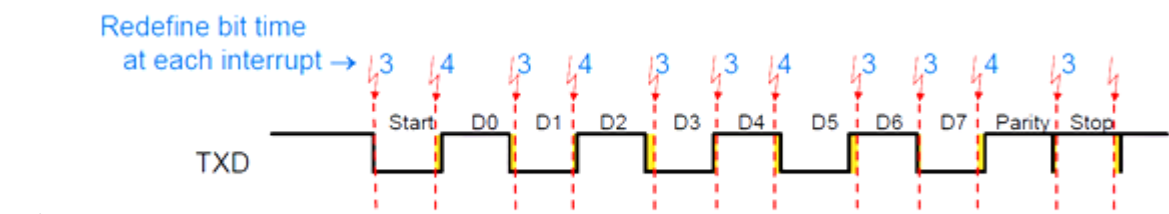
图 29-4：LPUART 发送时序图
