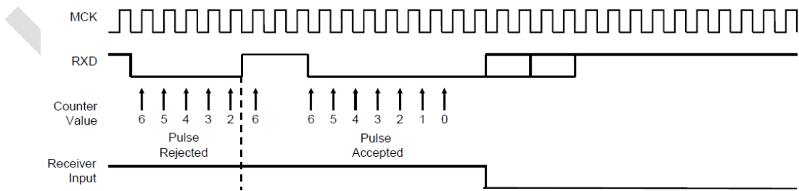
图 30-26: IrDA 解调器操作
