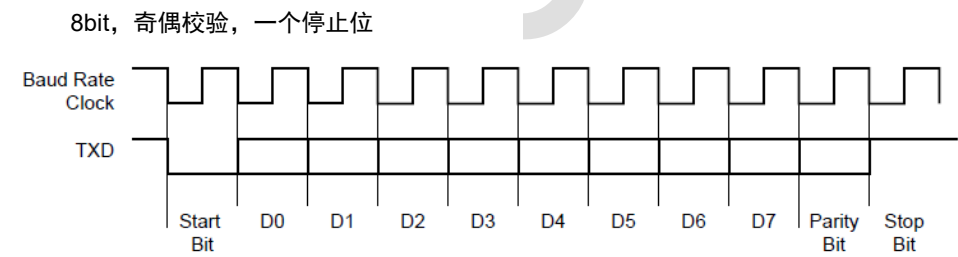
图 30-1: USART 字符发送
