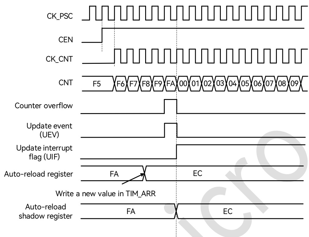
图 19-7: ARPE=1 (TIM_ARR 预装载) 时的更新事件
