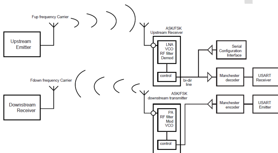
图 30-12: 曼彻斯特编码字符射频传输图
