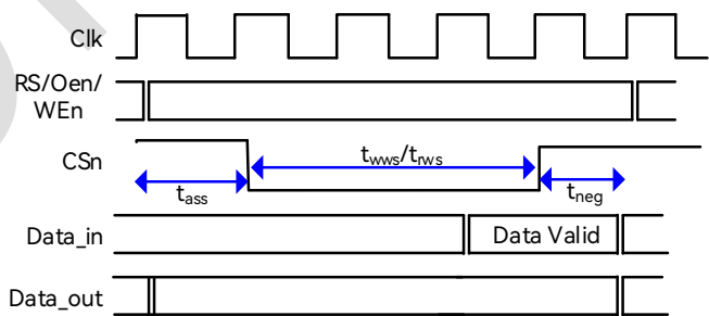
图 13-3: I8080 TFT-LCD 时序接口
