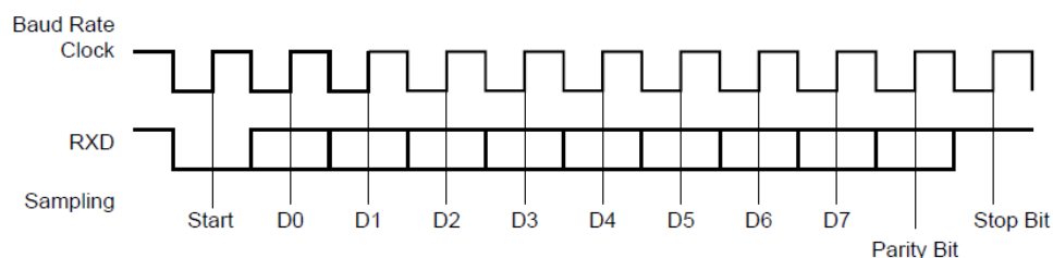
图 30-15: 同步模式字符接收
