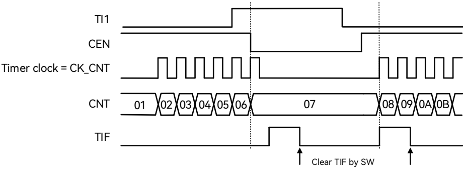
图 19-34: 门控模式下的时序
