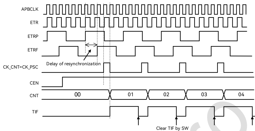
图 19-21：外部时钟模式 2 下的时序 2
