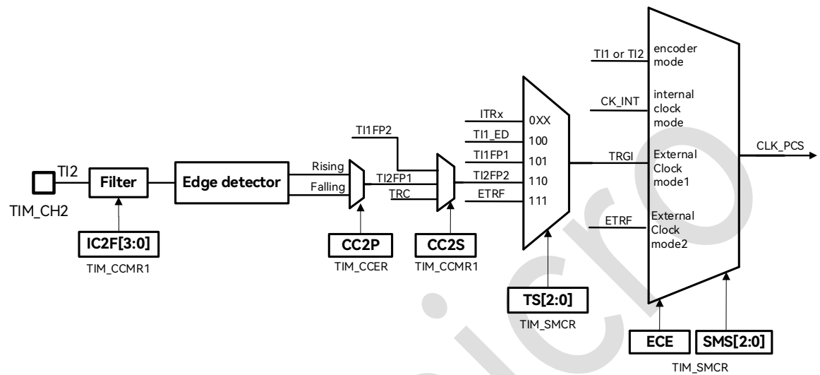
图 18-17：外部时钟连接图
