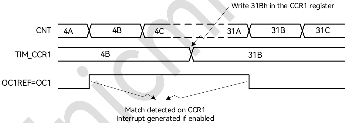
图 18-28：输出比较模式，翻转 OC1 时序图
