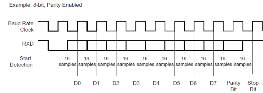
图 30-8：字符接收
