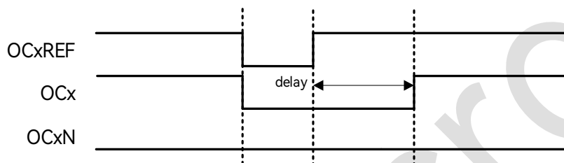
图 18-32: 死区波形延迟大于负脉冲时序图
