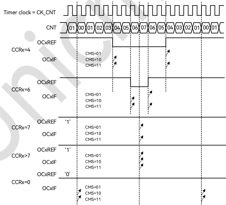
图 19-29: 中央对齐的 PWM 波形 (ARR=7)
