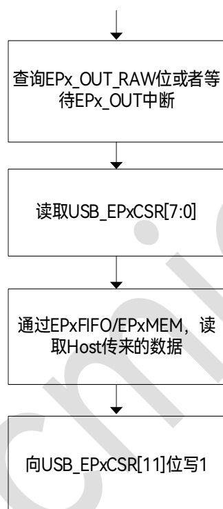
图 35-3: USB Endpoint Out 传输流程图
