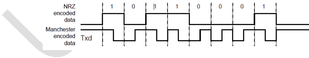
图 30-3: NRZ 码转为曼彻斯特码
