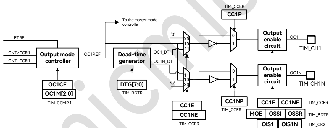
图 18-25: 捕获/比较通道的输出部分（通道 1 至 3）图
