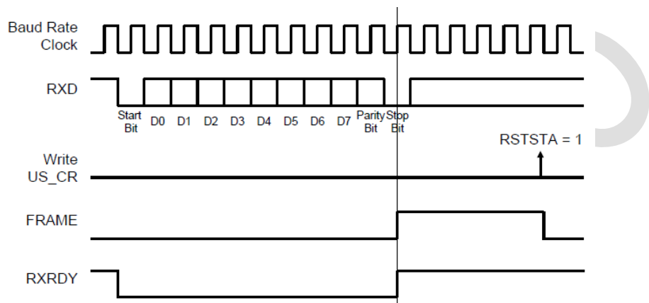
图 30-19：帧错误状态时序图
