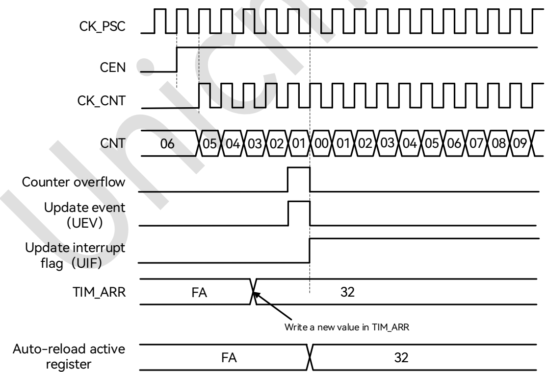
图 18-13: 计数器时序图, ARPE=1 时的更新事件 (计数器下溢)
