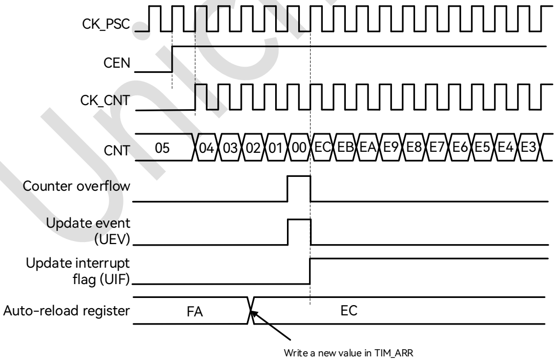
图 19-11: 向下计数，不使用重复计数时的更新事件
