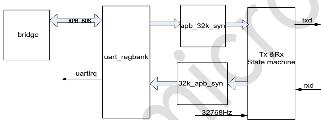
图 29-1：LPUART 结构框图
